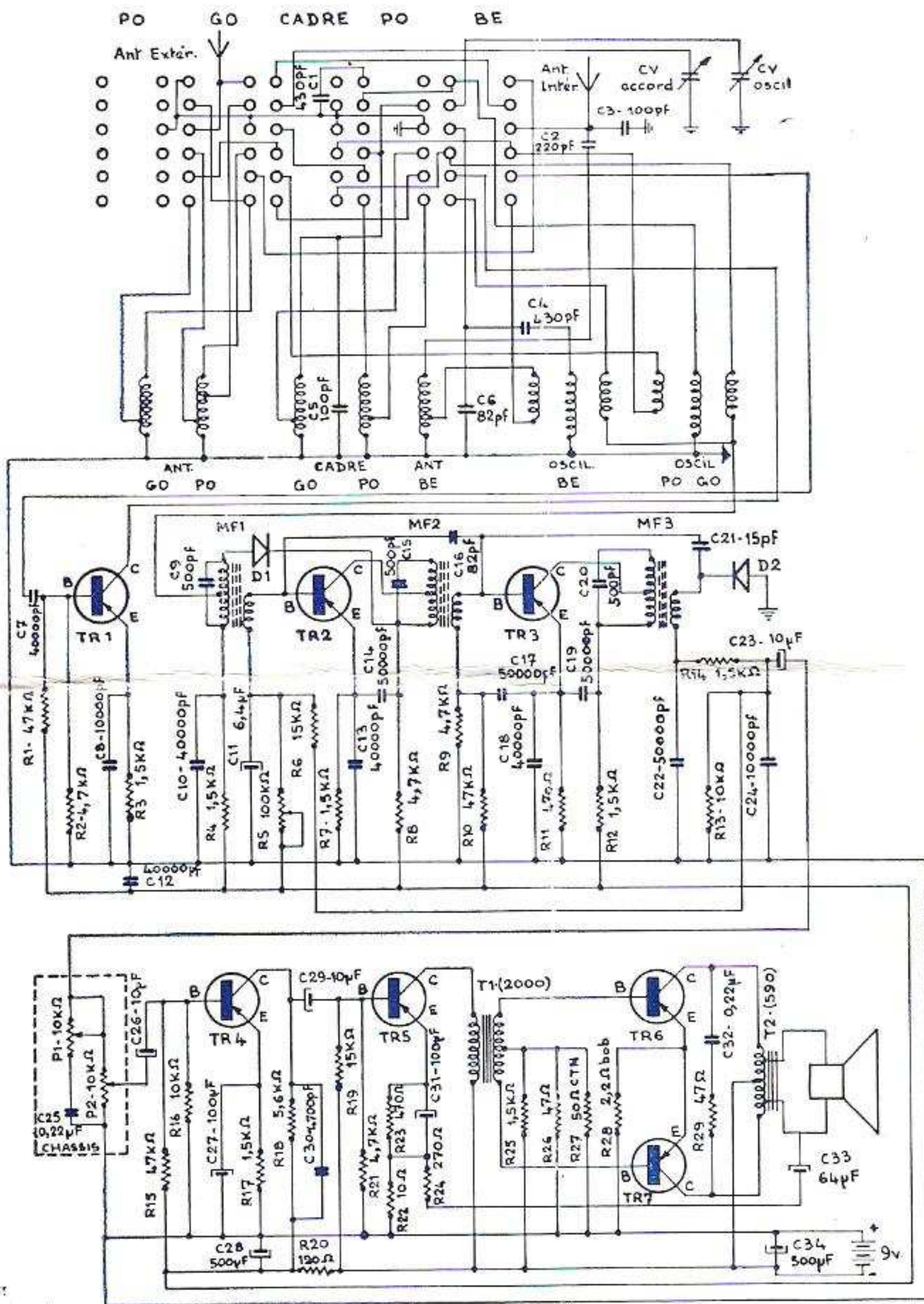
Schéma du Translitor 750
