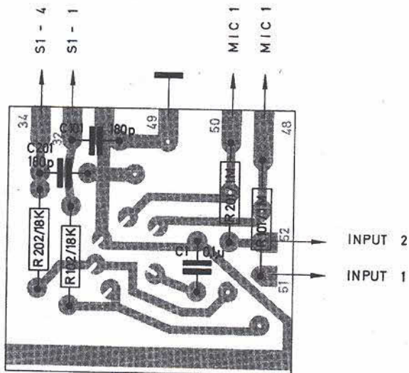
Fig. 14 Ätzschatplatte kpl. für Rückwand Europa (Leiterseite) 220 617
