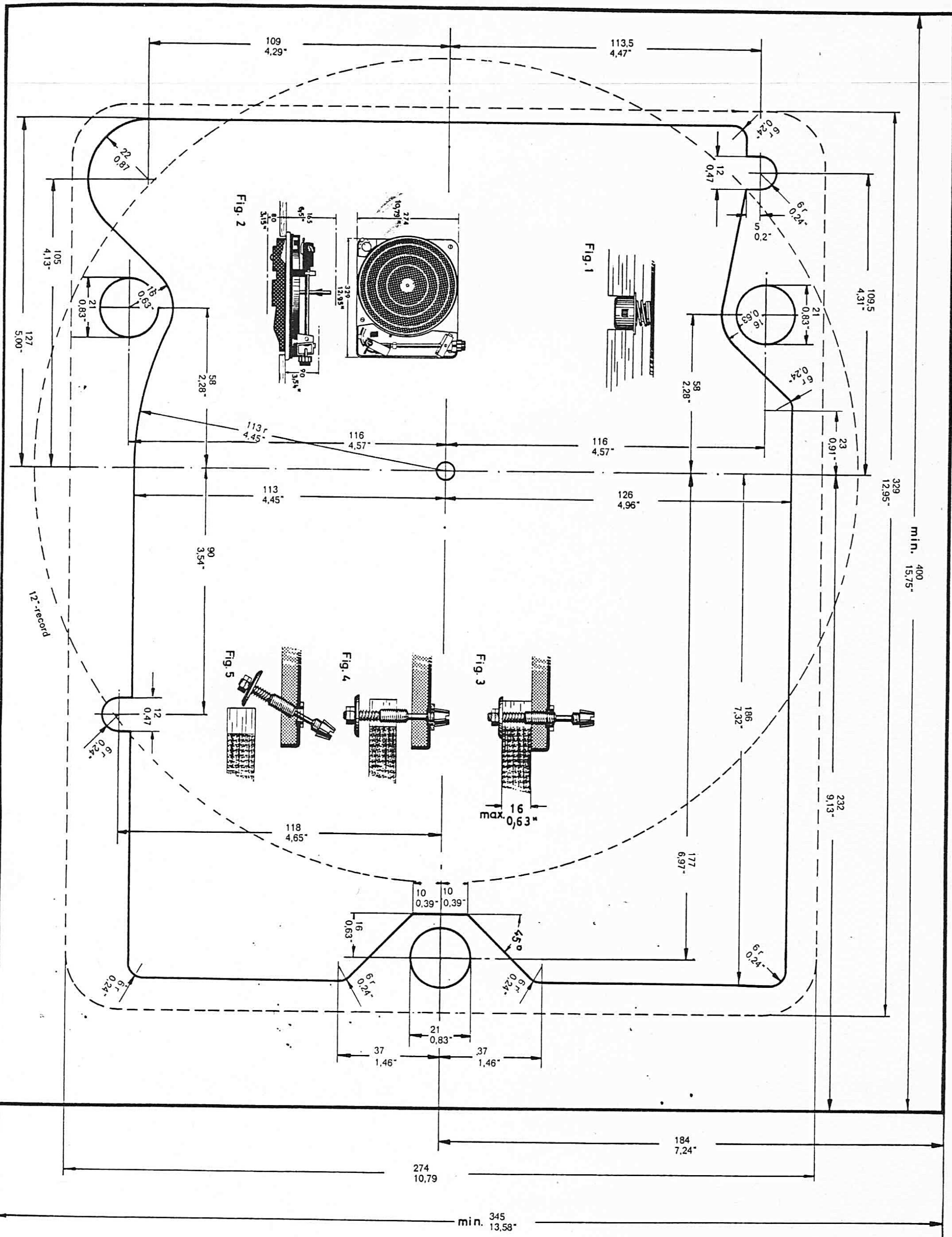
Abb. 14, Einbauschablone
