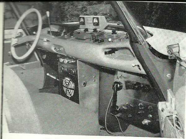
DS 19 avec Ampex 600
