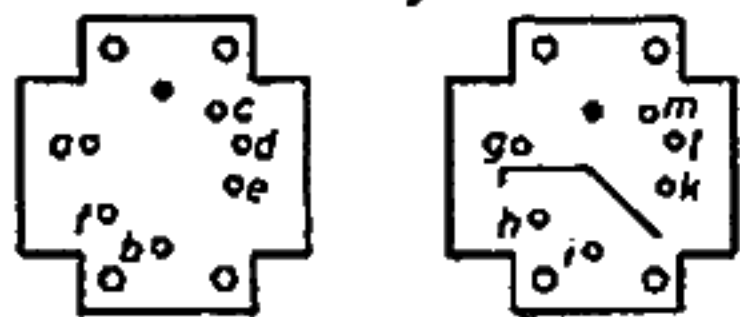
Kontaktplatte für GRUNDIG Hi Fi - Strahler Fern - Dirigent (von innen gesehen)
