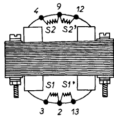
Transformateur d'origine
