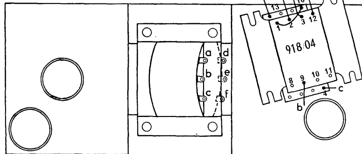
Transformateur standard A9 999 18/04
