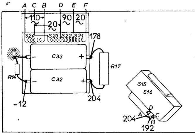
Caractéristiques électriques et commutations du transformateur d'alimentation FD 040 48
