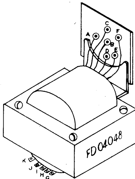
Transformateur d'alimentation FD 040 48
