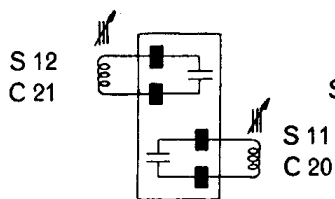
Filtre MF 1 FK 853 17
