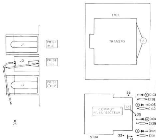
PLATINE ALIMENTATION (côté éléments)
