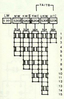
SCHALTERDIAGRAMM VON BESTÜCKUNGSSEITE AUS GESEHEN
