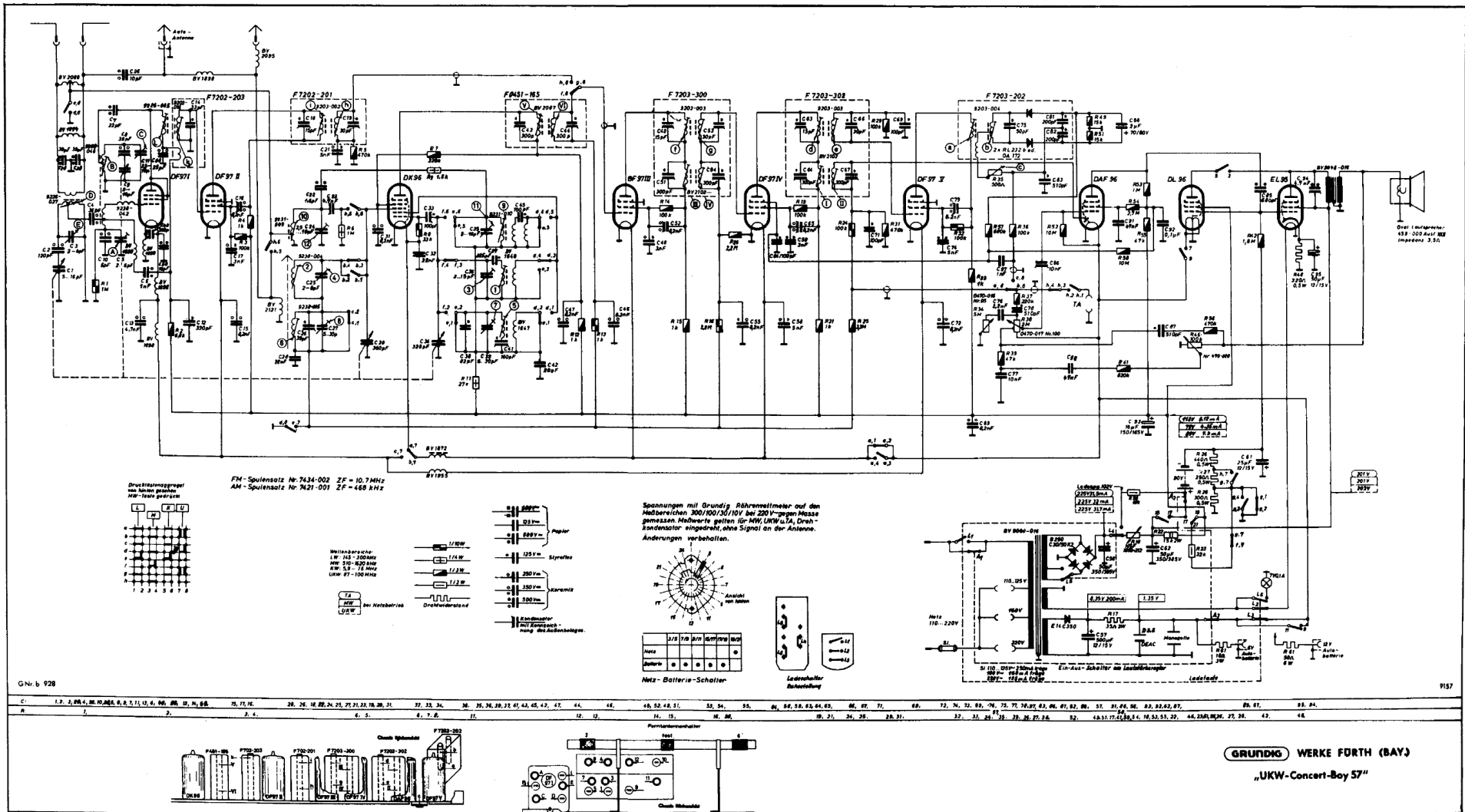
GRUNDIG (Radio Werke Fürth/Bay) - Mod. UKW-Concert-Boy 57. Apparechio portatile del tipo a modulazione d'ampiezza e di frequenza. Gamme d'onde lunghe, medie, corte e ultracorte (FM). Medie frequenze a 468 kc e a 10,7 Mc/s. Alimentazione con pile a secco incorporate, dalla batteria d'accumulatori o con tensione alternata della rete-luce.
