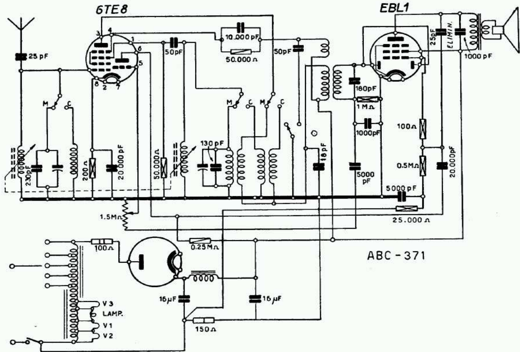
ABC RADIO - Mod. 371 - Supereterodina gamma onde medie. Valvola 6TE8 convertitrice di frequenza con exodo, e preamplificatrice BF con triodo. Valvola EBL1 rivelatrice e amplificatrice finale. Sintonia ad induttori variabili. Media frequenza 465 kc.
