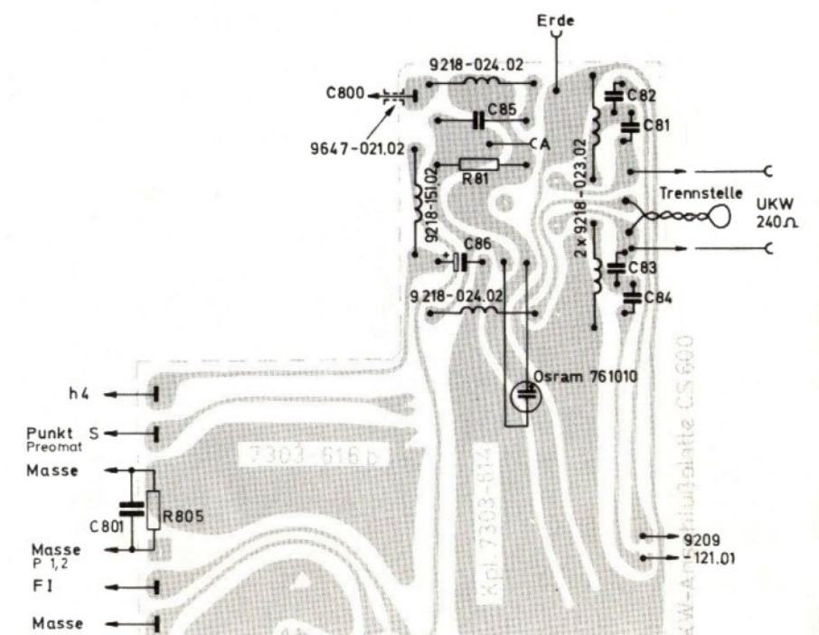
Bloc, vu du côté des composants
