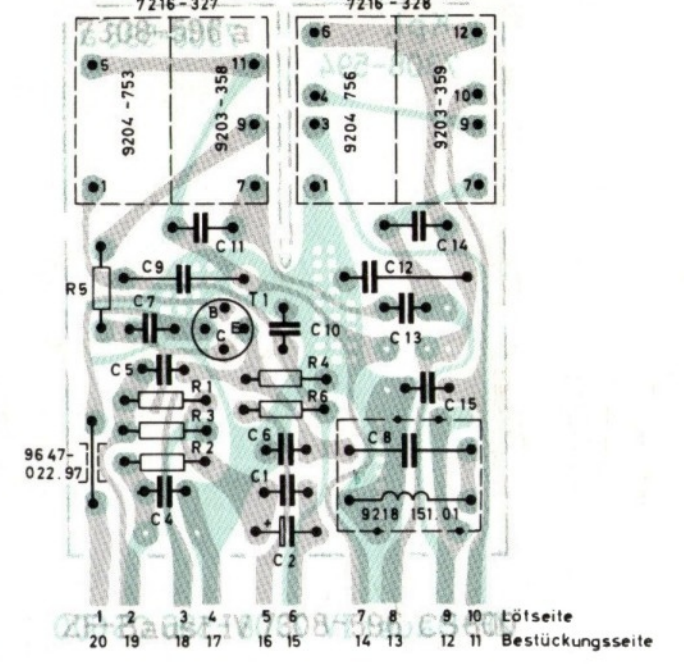
Plaque 56 V, vu du côté des soudures
