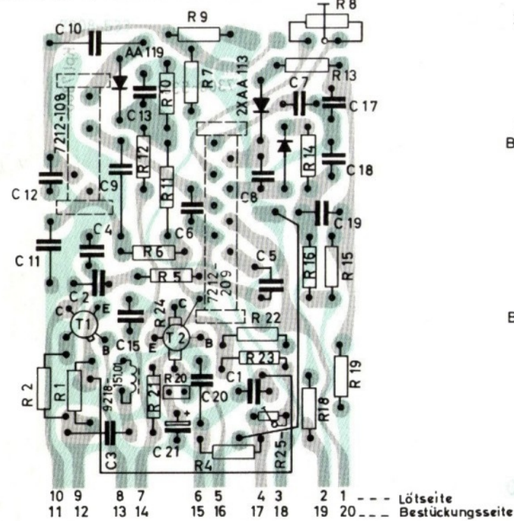
Plaque de connexion FM, vu du côté des soudures
