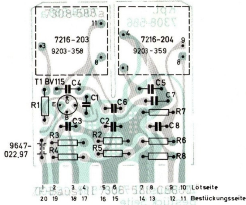
Filtre FI II, vu du côté des soudures
