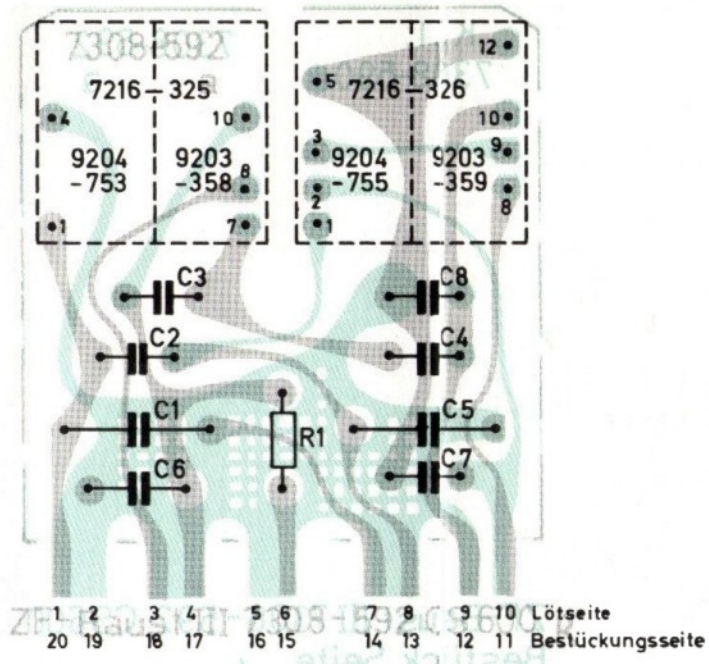
Filtre FI III, vu du côté des soudures
