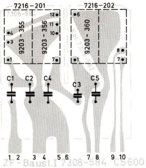
Filtre FI V, vu du côté des soudures
