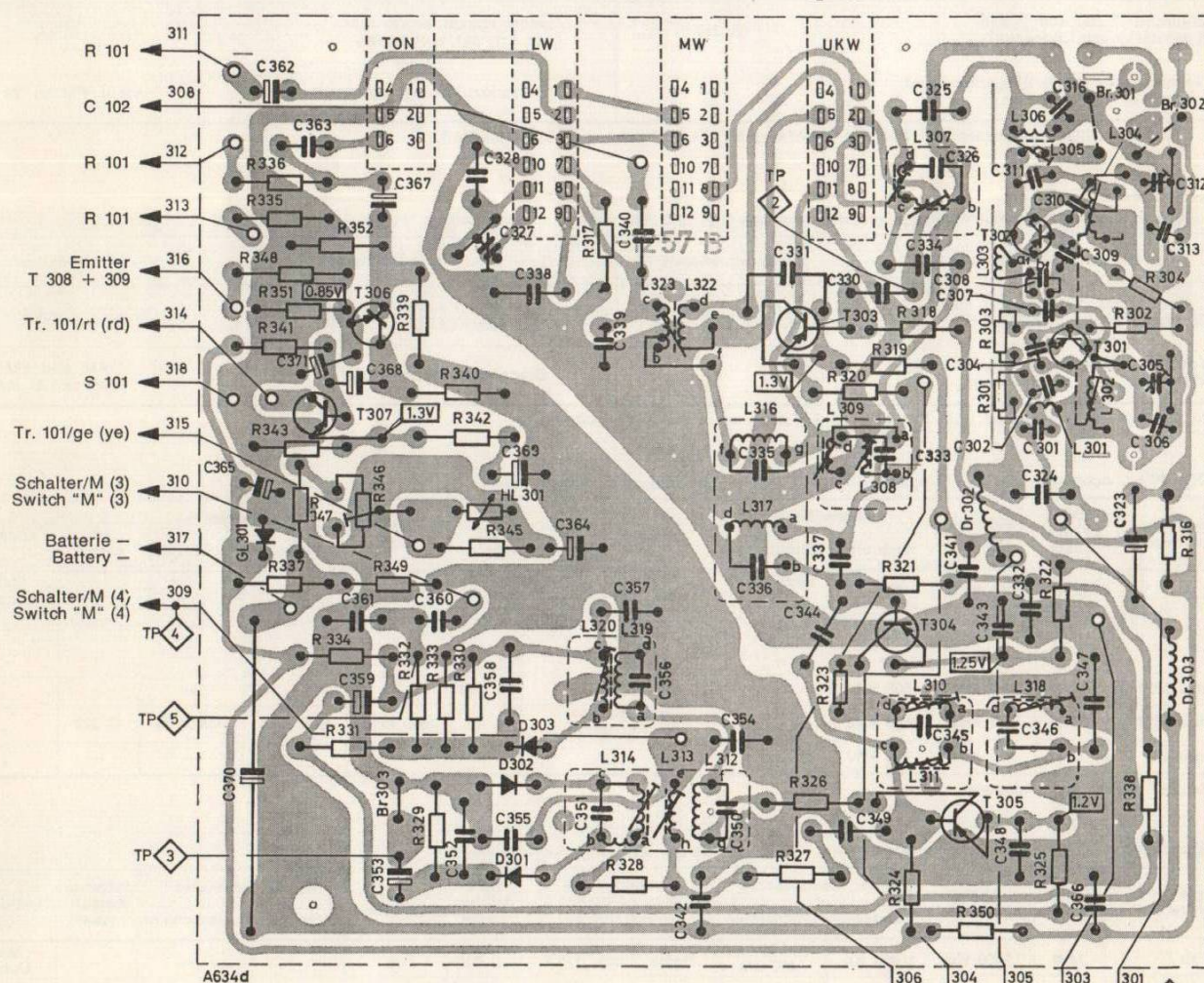
Gedruckte Schaltung – Verdrahtungsseite Printed Circuit – Wiring Side
