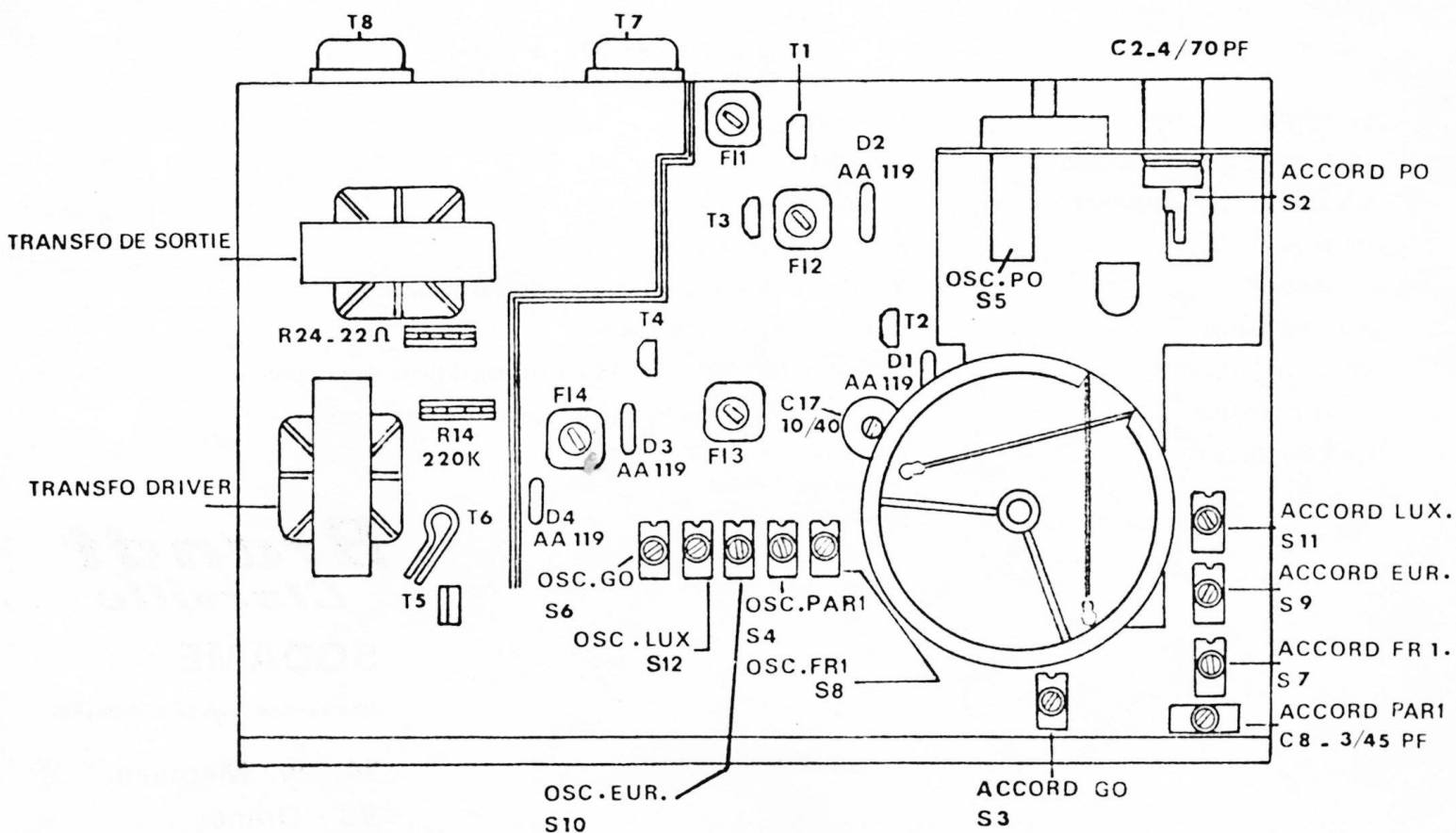
VUE DE DESSUS DES PRINCIPAUX ELEMENTS
