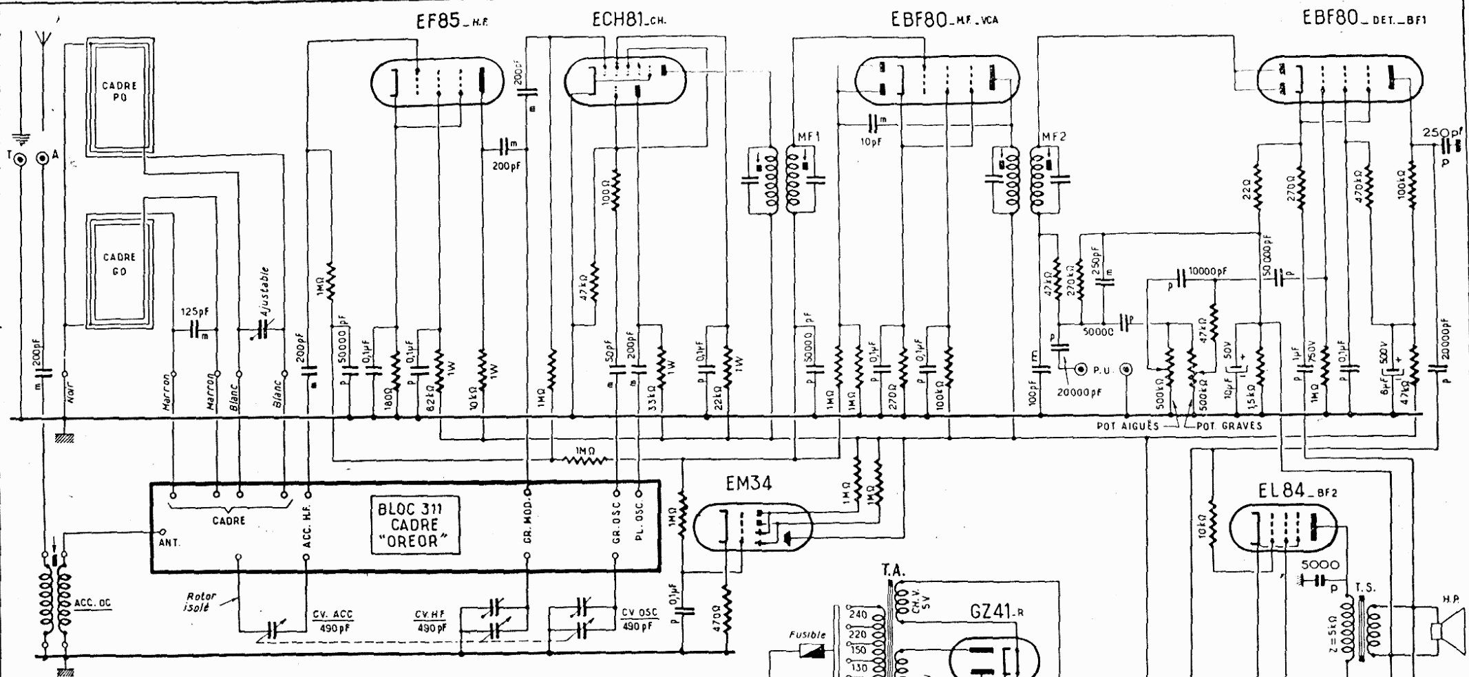
RÉCEPTEUR ANTIPARASITES 7 TUBES CADRE H.F. ACCORDÉ ET COMPENSÉ - TUBES NOVAL MÉLANGEUR GRAVES ET AIGÜES - CONTRE-RÉACTION B.F.
