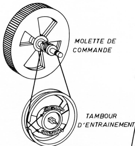
DETAIL DU MONTAGE
