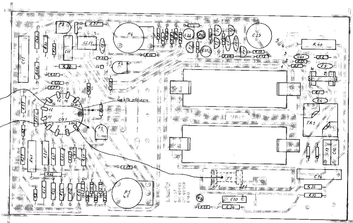
EMO 500 - schéma d'implantation
