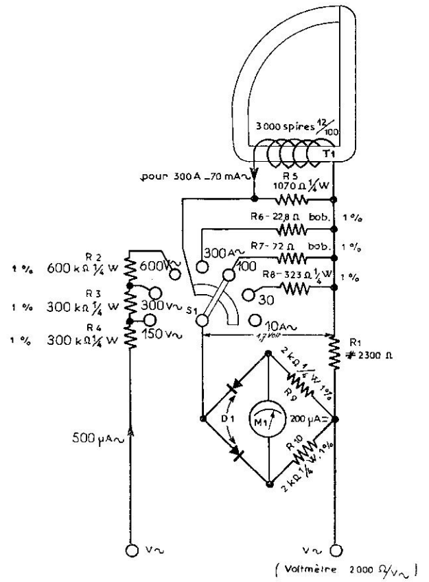
ELECTROPINCE 400 : SCHEMA DE PRINCIPE
