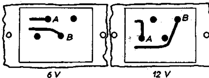
Sous le couvercle du transformateur du vibreur
