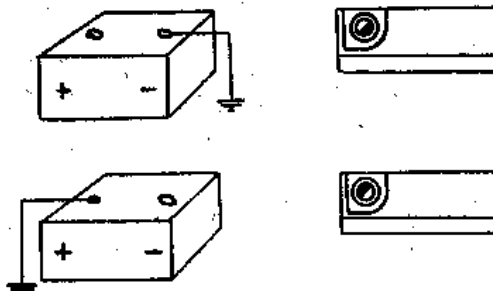
Position du vibreur selon la polarité de la batterie
