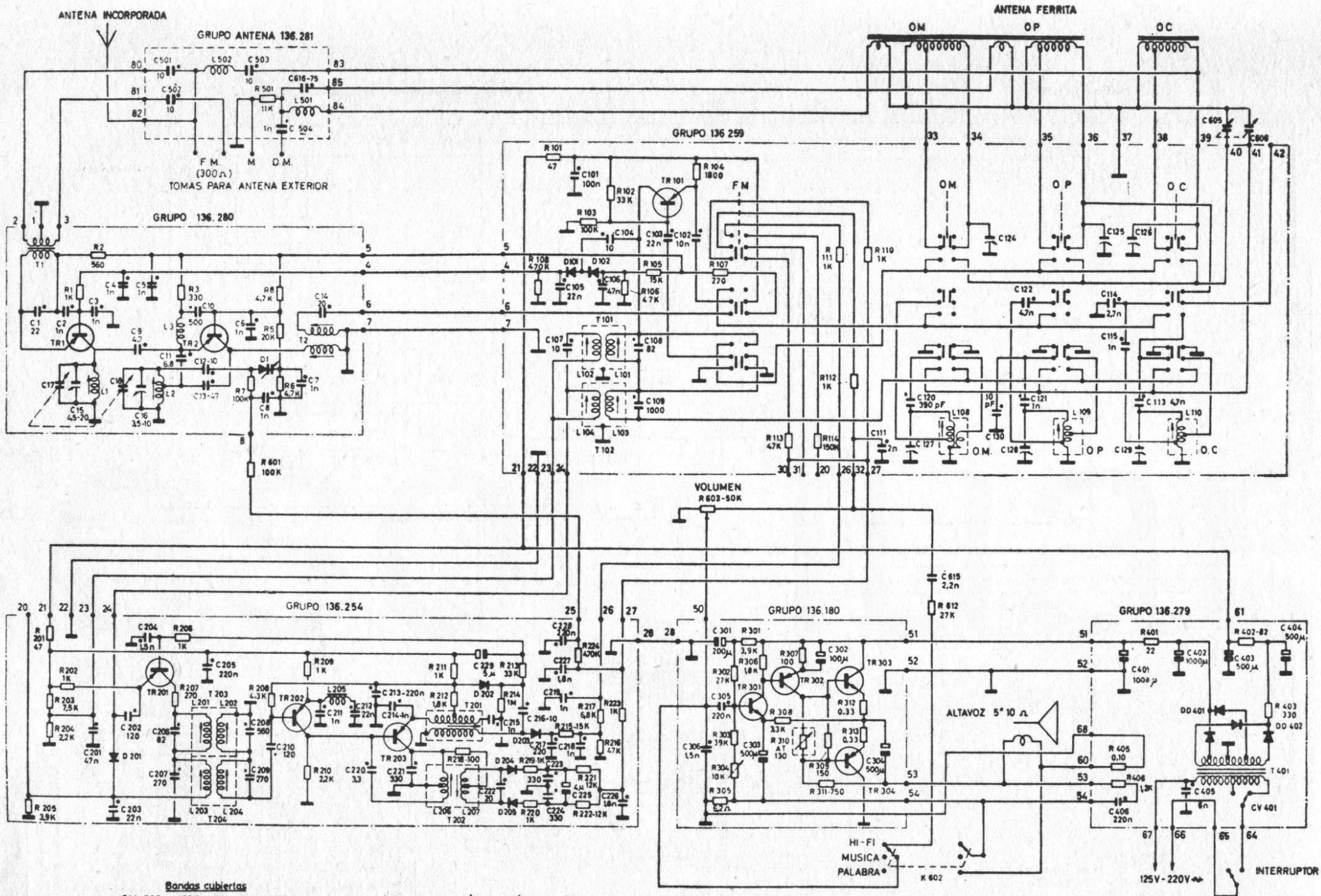
INTER Modelo "Euromodul 101 / FM"
