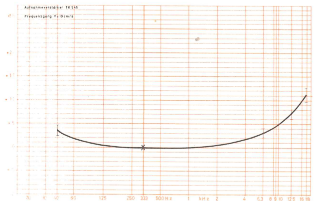
Abb. 15 Frequenzkurve „Aufnahme 19 cm/s“
