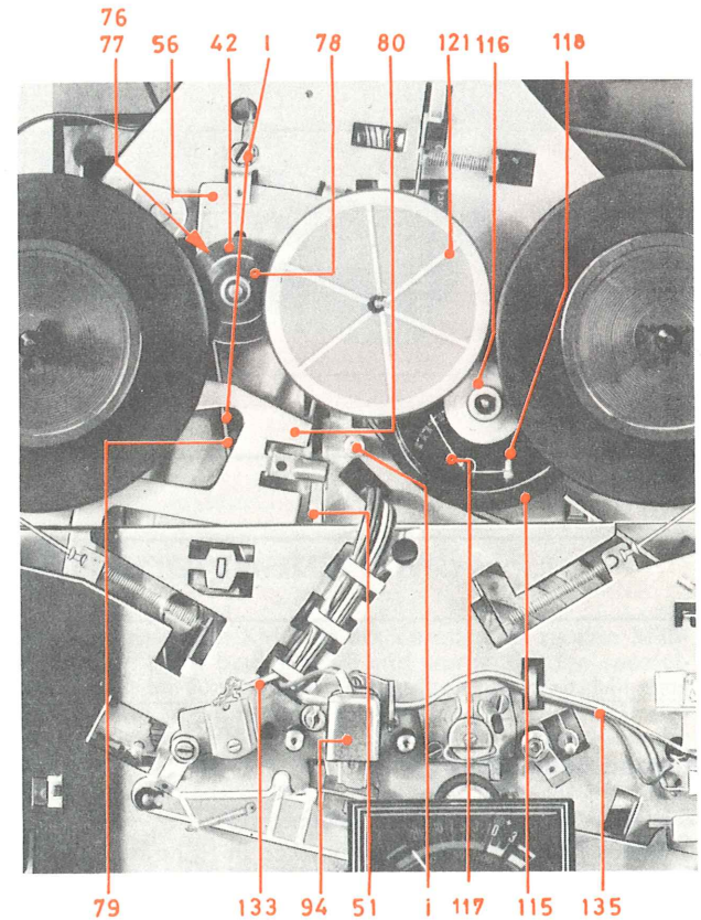
Abb. 6 Riemenwechsel/Aufwickelkupplung
