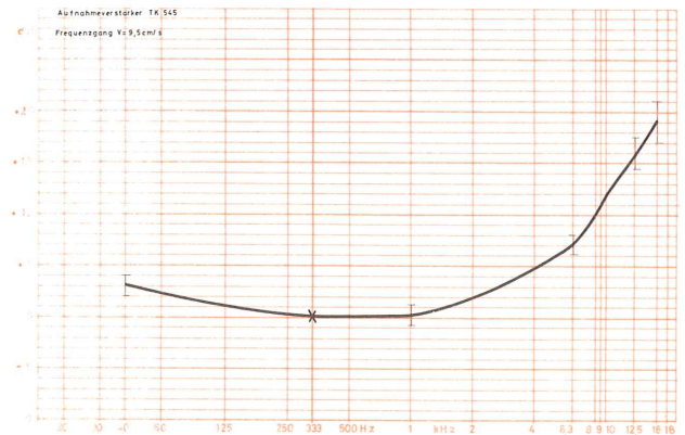
Abb. 14 Frequenzkurve „Aufnahme 9,5 cm/s“
