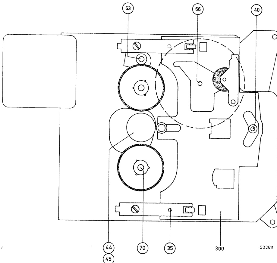
Fig. 10—Lubrication Chart
