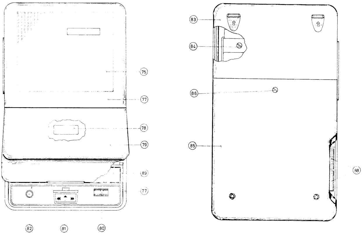
Fig. 2—Cabinet View—ST473
