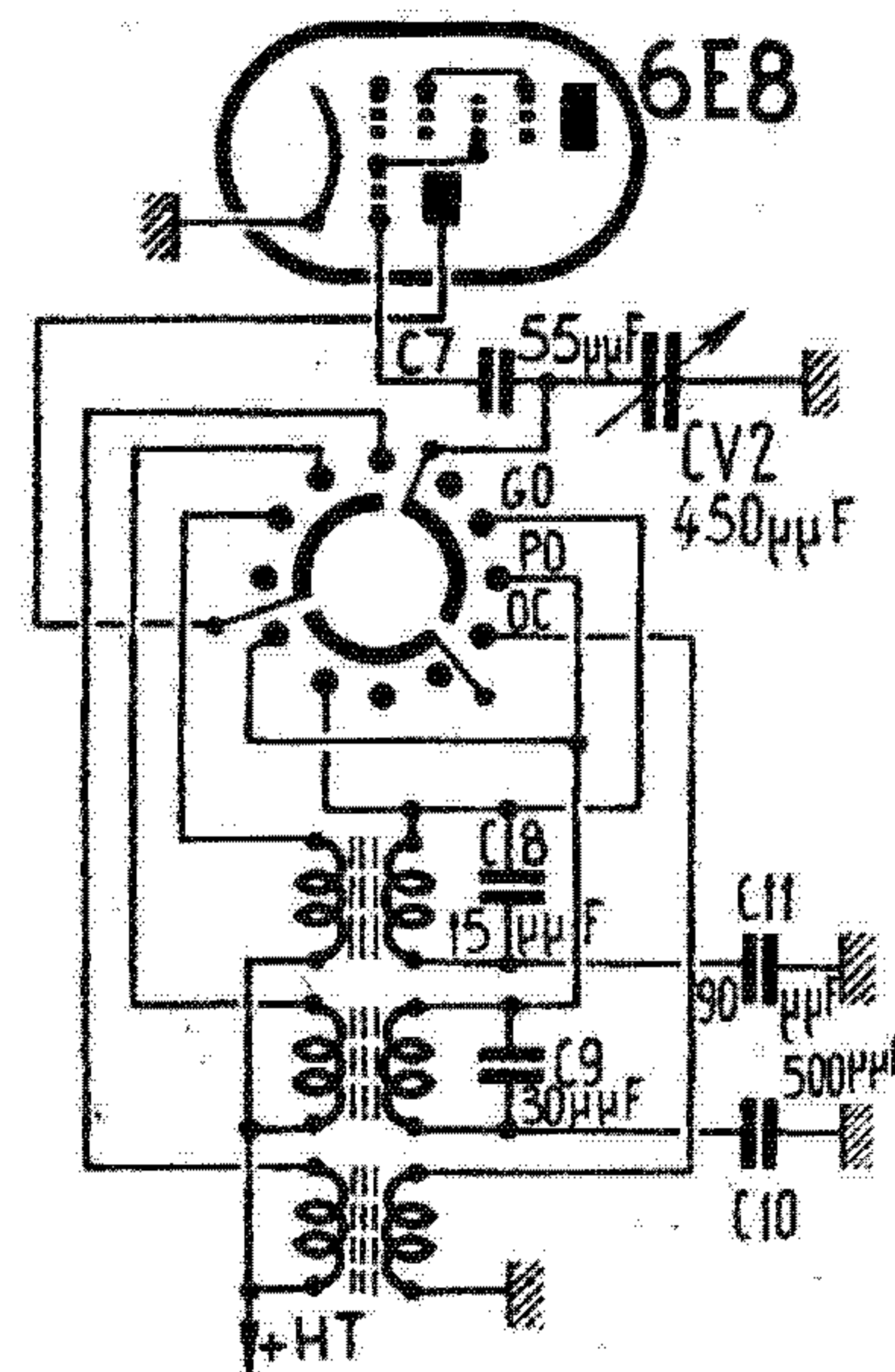
Montage avec grille accordée
