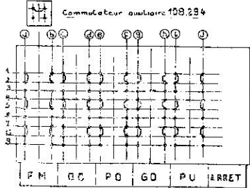
Schema du commutateur à cliquer ou de l'intérieur du chassis. Les contacts sont représentés dans la position repos.
