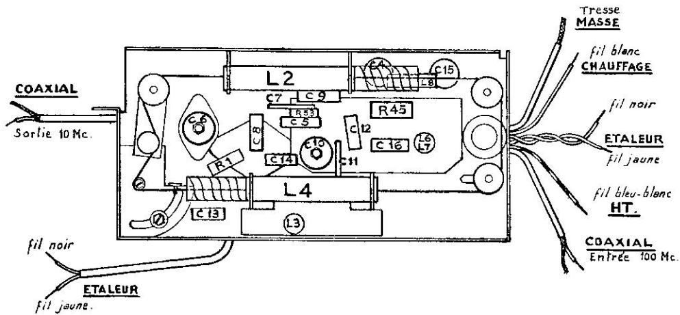
VUE INTÉRIURE
