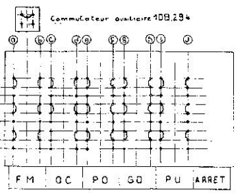
Schema du contacteur à placer au de l'intérieur du chassis. Les contacts sont représentés dans la position repos.
