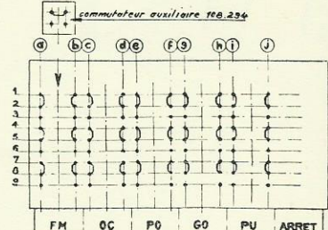
Schema du contacteur à levier, vu de l'intérieur du chassis. Nota: Les contacts sont représentés dans la position repos.
