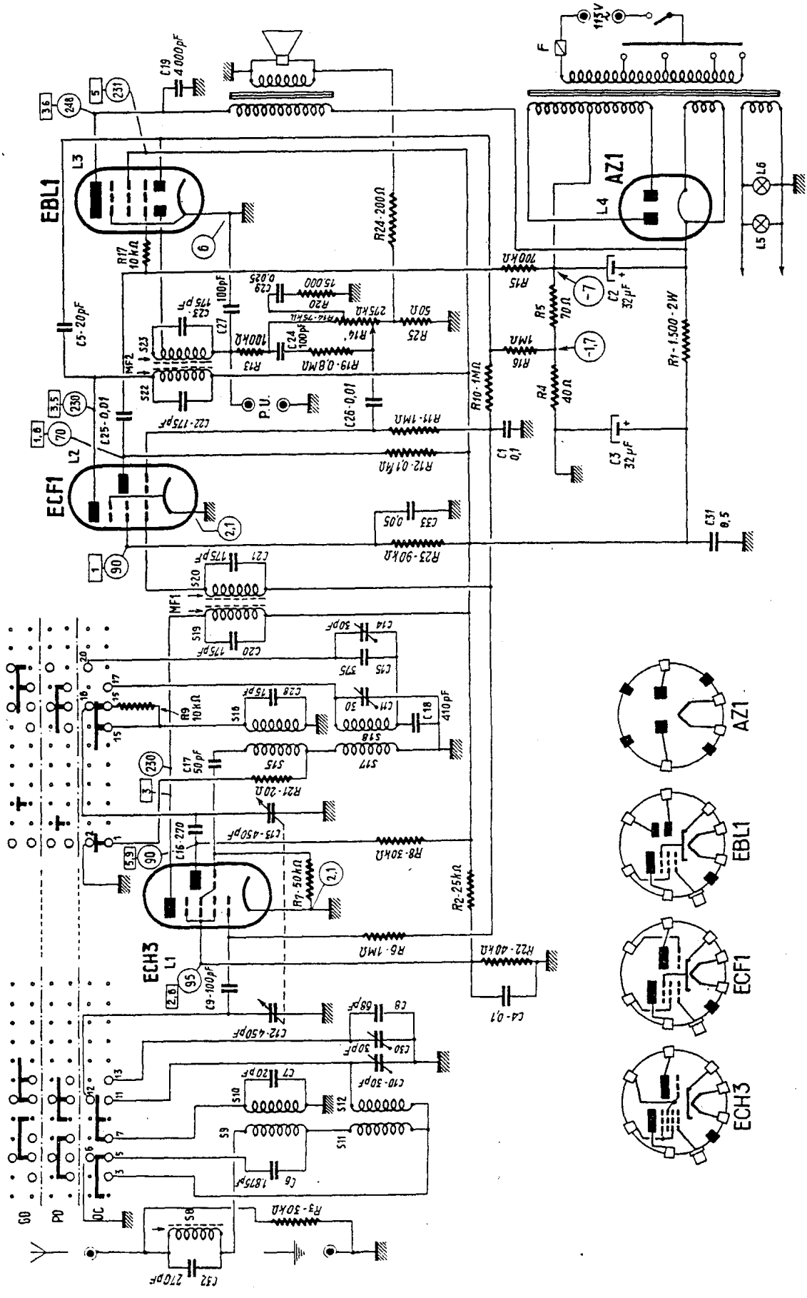
Schéma général complet des récepteurs Philips BF371A et Radiola RA73A
