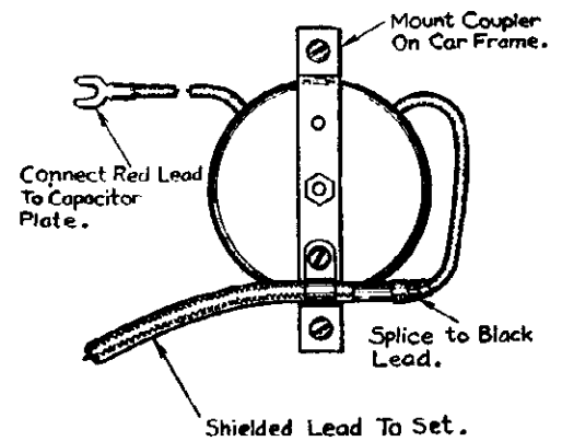
Fig. 6—Coupler.
