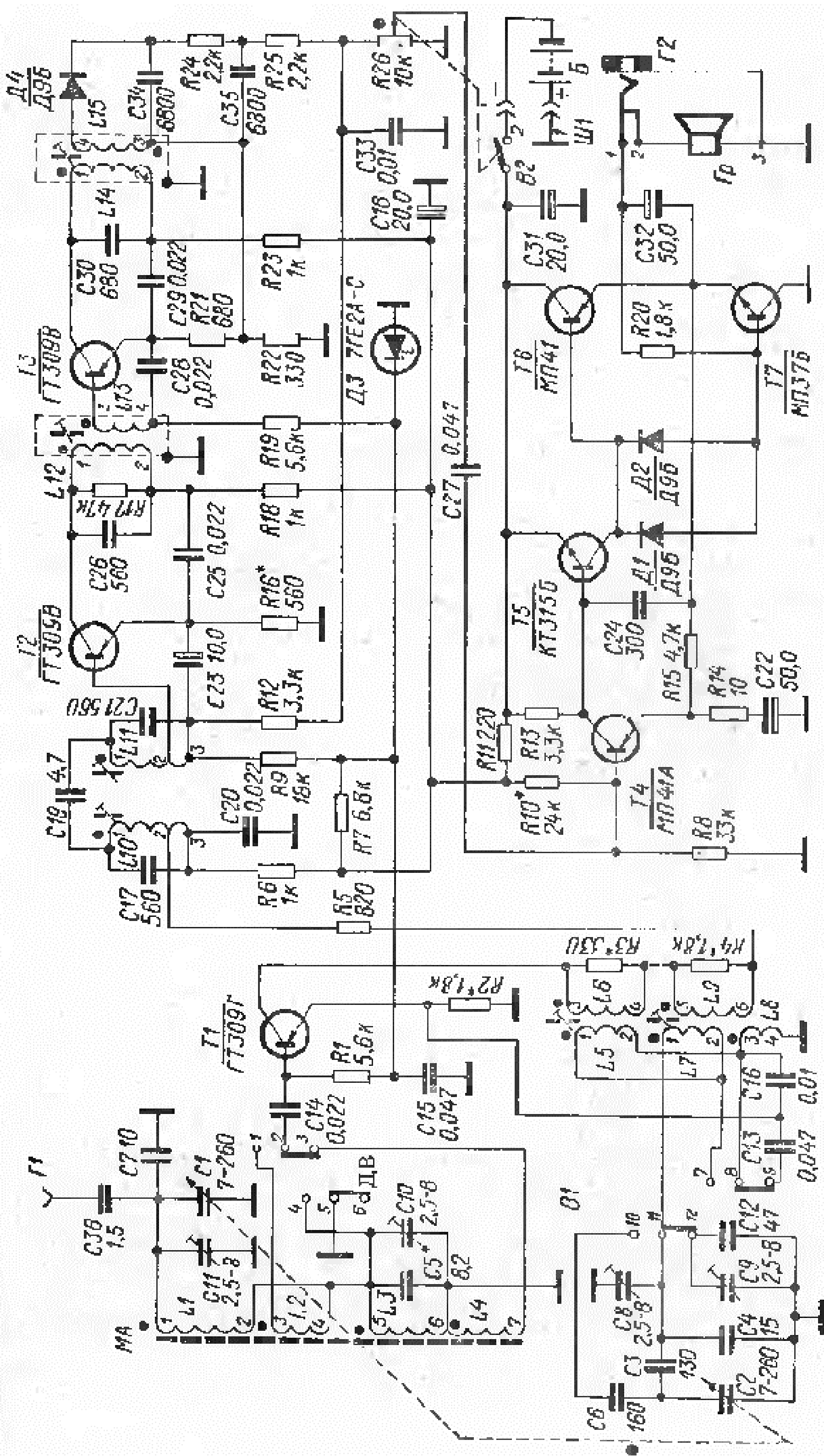
Рис. 12. Принципиальная схема радиоприемника «Этюд-2»
