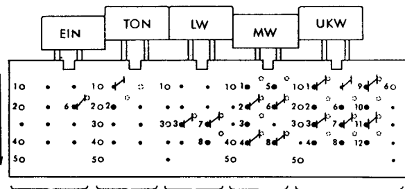
Kontaktplan, Stand MW- und Ein-Taste gedrückt, gesehen auf Printseite
