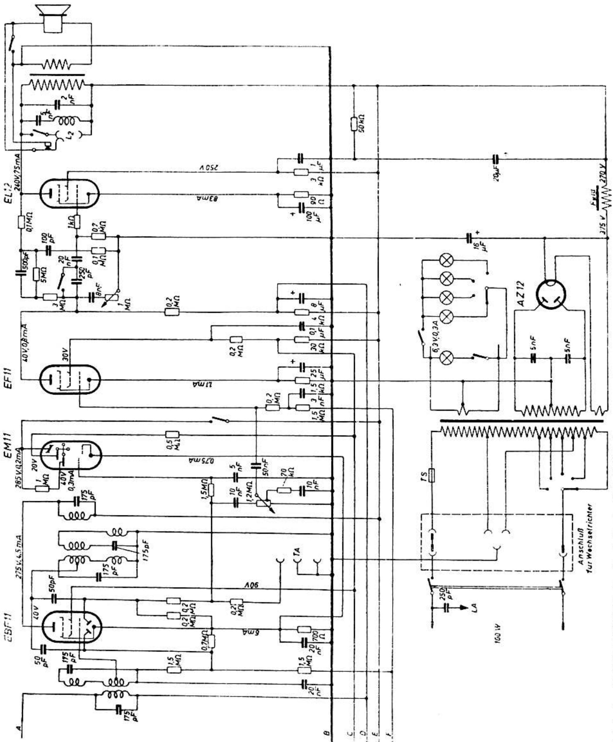
Telefunken D 860 WK/WKZ (rechte Seite des Schaltbildes)
