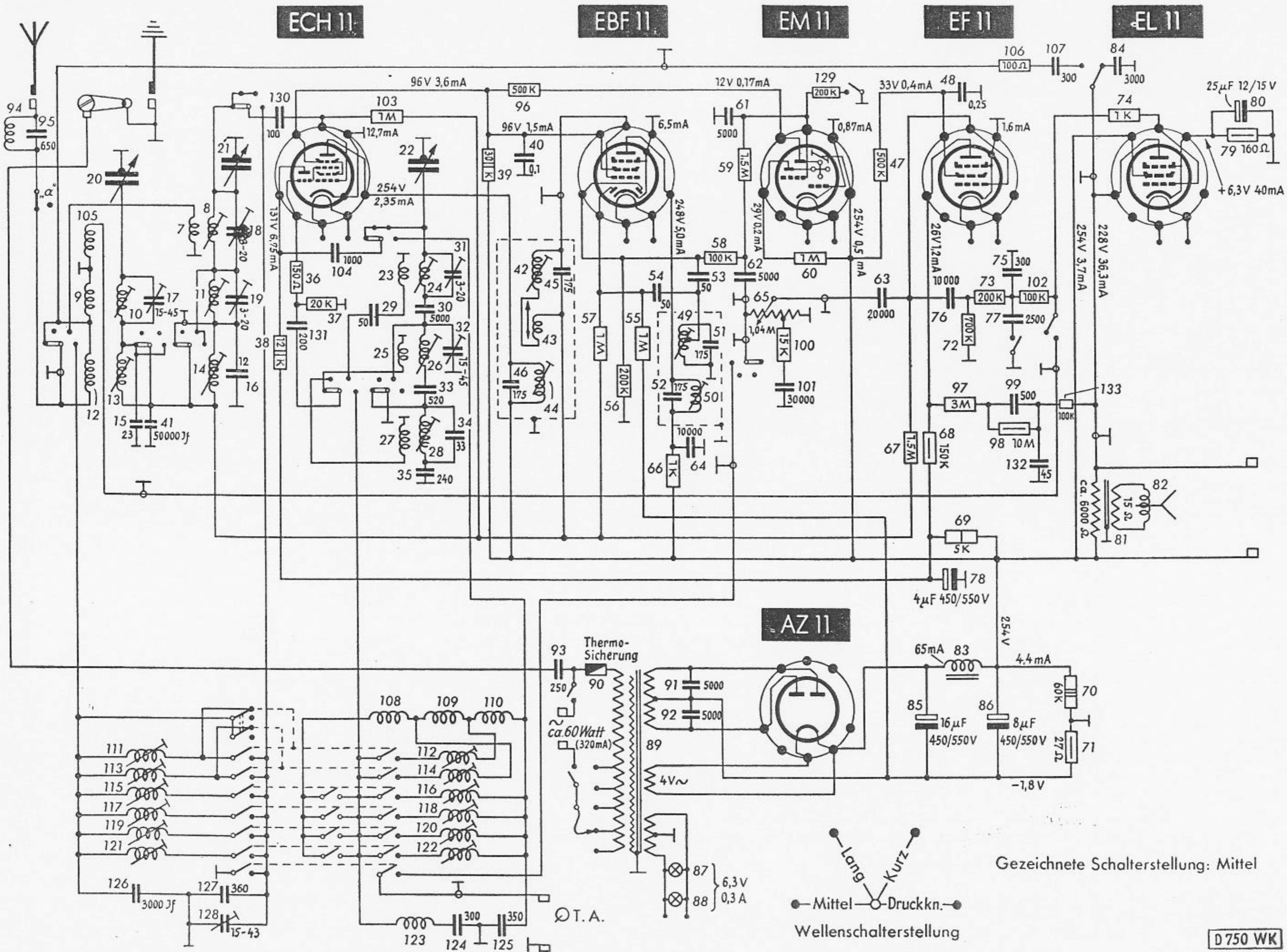
Schalbild
