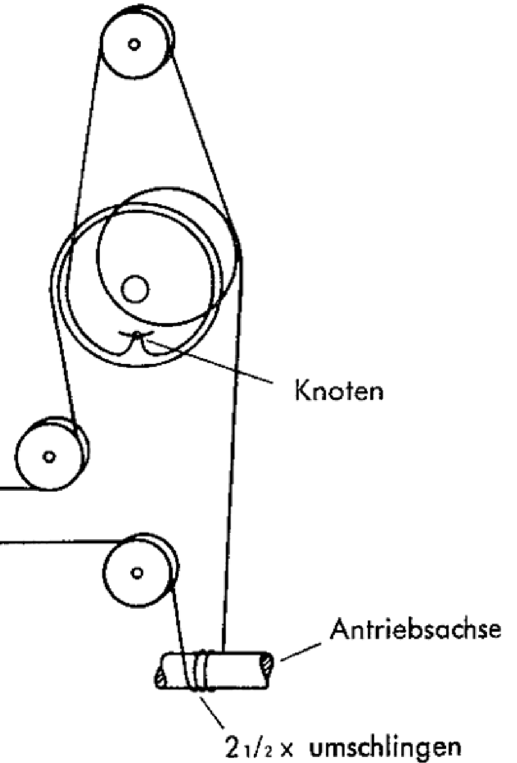
Schnurlaufführung bei Musikgerät 65 von vorne gesehen
