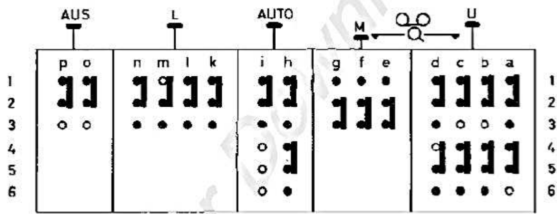
Schalterdiagramm / Switch diagram Gezeichnete Schalterstellung: M Switch shown in position: M
