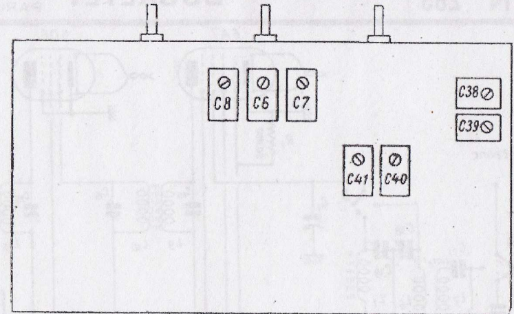
Disposition des ajustables à l'intérieur du châssis.
