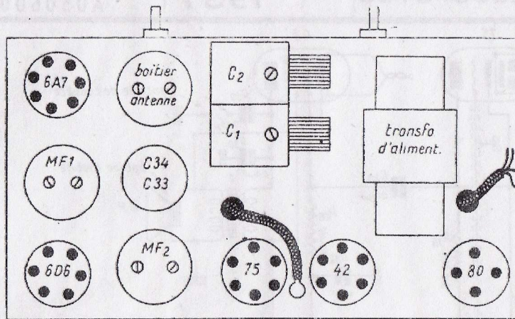
Dispositions des éléments sur le dessus du châssis.
