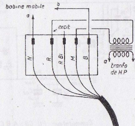
Branchement du H.P. avec indication de la couleur des fils.
