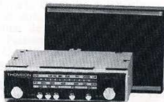
THOMSON DUCRETET Récepteur auto-radio
