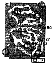
DÉTECTION Circuit vue côté cuivre
