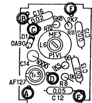
DÉTECTION Circuit vue côté éléments
