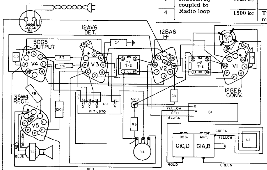
Fig. 7. Wiring Diagram
