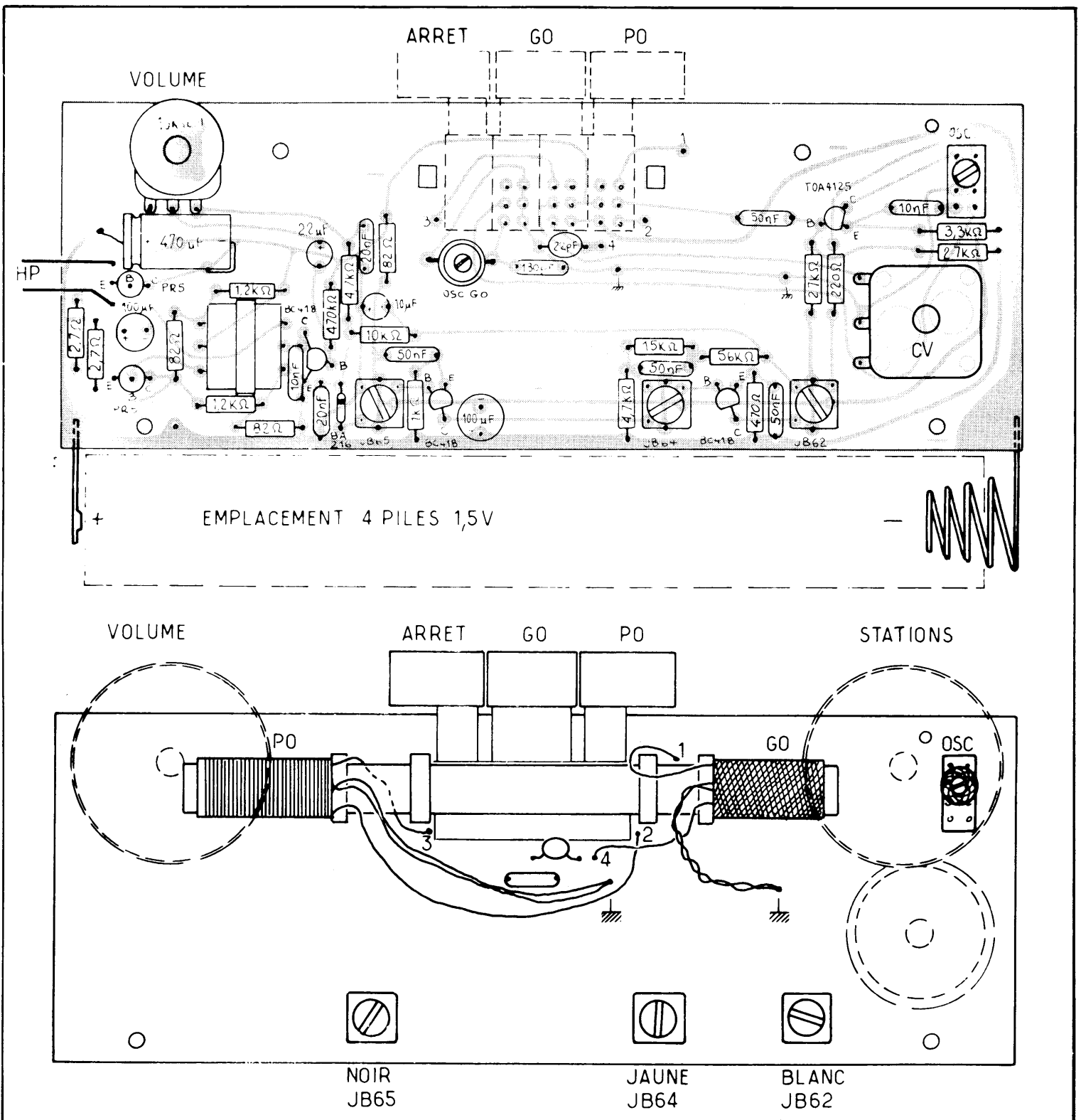
Fig. 2. et 3. - Comme il s'agit d'un ensemble commercialisé sous la forme de kit, c'est-à-dire en pièces détachées, dans un premier temps l'amateur aura à se livrer à la mise en place des composants sur le circuit imprimé entièrement préparé à cet effet.
