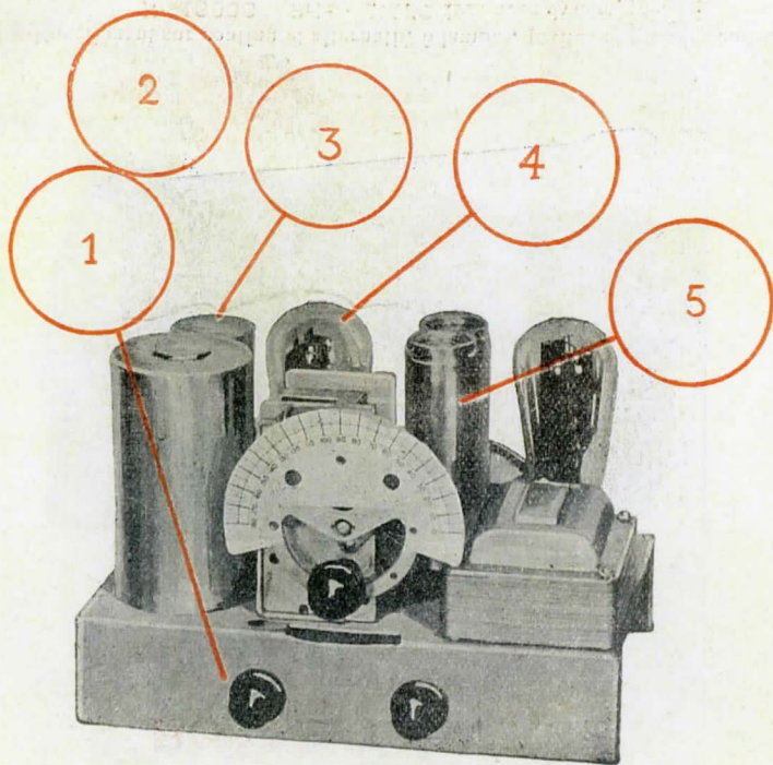
1. Circuit préselecteur ; 2. Dynamique licencié ; 3. Détectrice pénthode 4. Pénthode B.F. de puissance 7 W. ; 5. Double filtrage secteur. Bloc condensateur variable à air Wireless . Prise pick-up.
