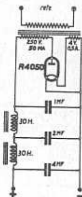
Alimentatore per apparecchi fino a 3 valvole
