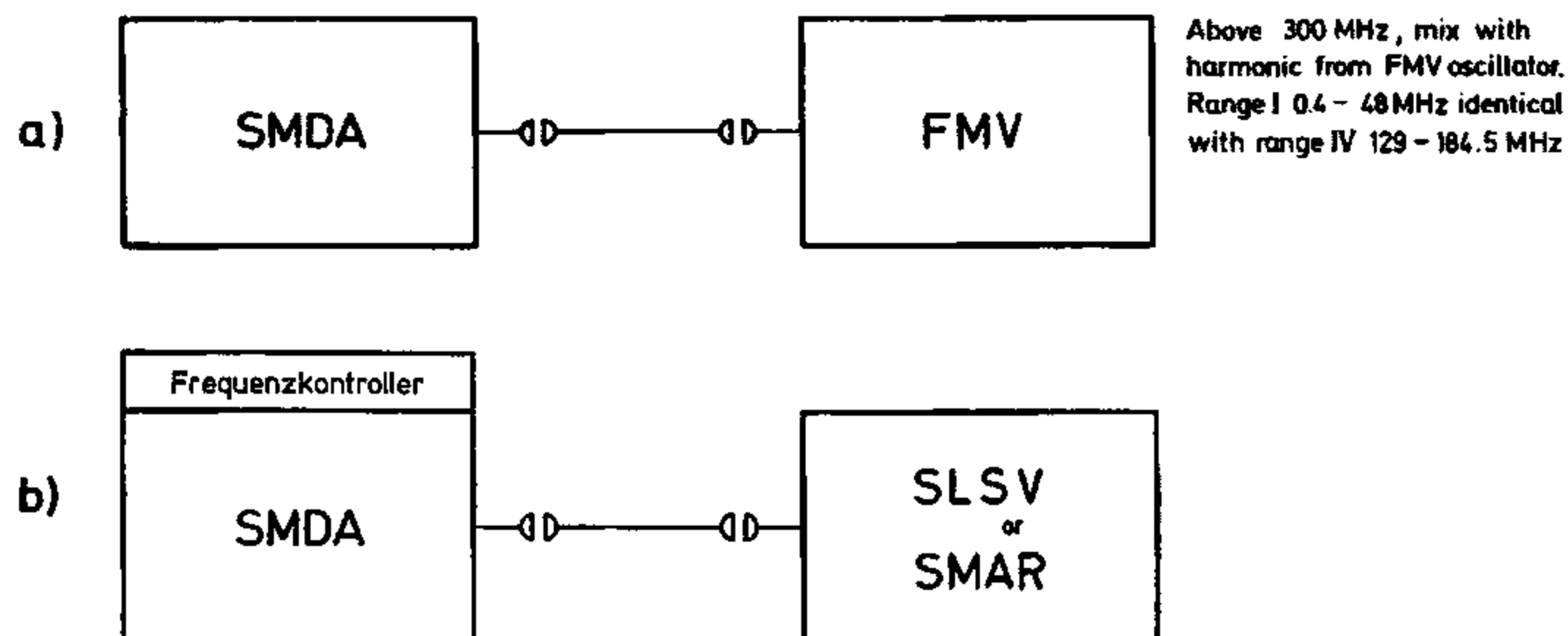
Fig. 3-15 Checking of internal FM und \phi M
