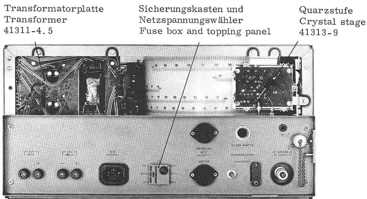
Bild 4-4 Ansicht von hinten ohne Kasten Fig. 4-4 Rear view, cabinet removed
