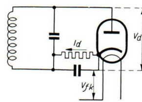
Définition de V_d et de I_d . Fig. 6
