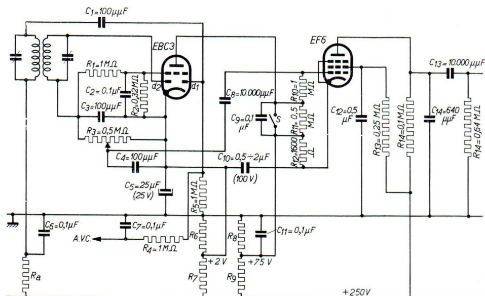
Montage de la lampe EBC 3 comme détectrice diode avec réglage silencieux. La lampe EF 6, montée en penthode ou en triode peut servir comme amplificatrice de basse fréquence. La diode d_1 est utilisée pour le réglage automatique différé du volume sonore.
