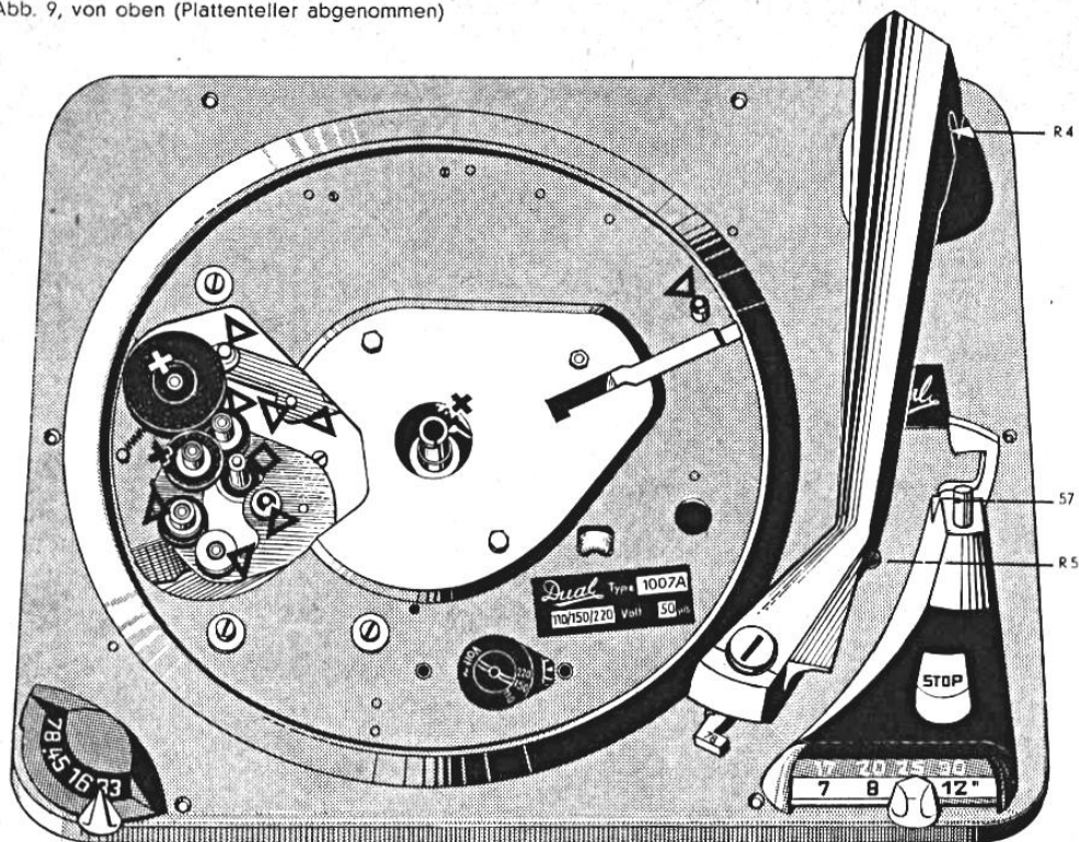
Abb. 9, von oben (Plattenteller abgenommen)
