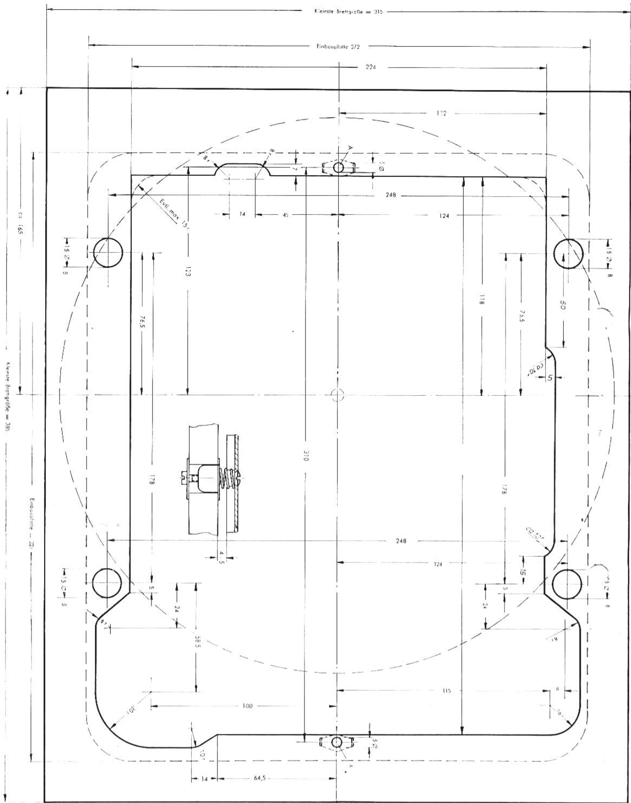
Abb. 13, Einbauschablone
