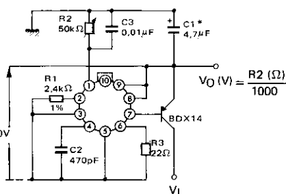
UTILISATION AVEC SOURCE DE POLARISATION EXTERIEURE OPERATING WITH SEPARATE BIAS SUPPLY
