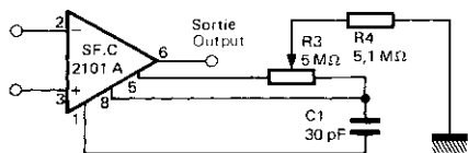
CIRCUIT D'EQUILIBRAGE BALANCING CIRCUIT
