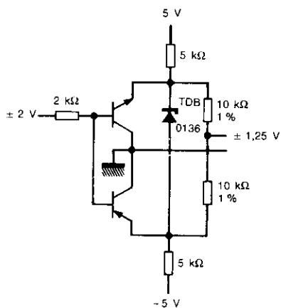
Figure 9. Source de référence bipolaire Bipolar output reference
