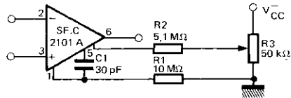
AUTRE CIRCUIT D'EQUILIBRAGE ALTERNATE BALANCING CIRCUIT
