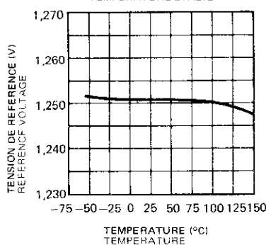
STABILITÉ EN TEMPERATURE TEMPERATURE STABILITY
