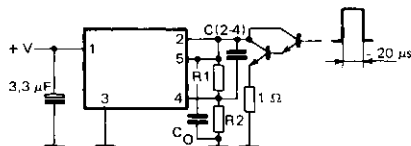
Fig. 17 - CIRCUIT DE MESURE EN IMPULSION TEST CIRCUIT FOR PULSE MEASUREMENTS
