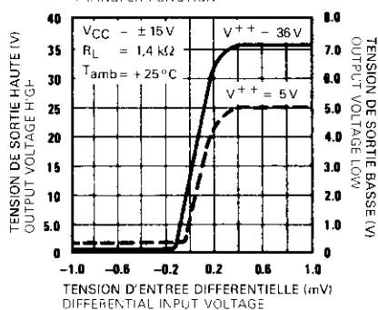
CARACTERISTIQUES DE TRANSFERT TRANSFER FUNCTION
