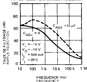
TAUX DE FILTRAGE EN FONCTION DE LA FREQUENCE RIPPLE REJECTION VERSUS FREQUENCY
