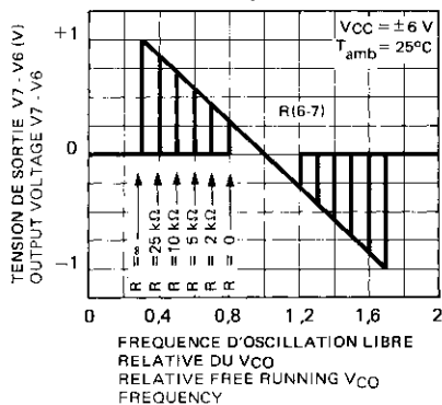
FIG. 7 — PLAGE DE VERROUILLAGE
