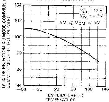
TAUX DE REJECTION EN MODE COMMUN COMMON MODE REJECTION RATIO
