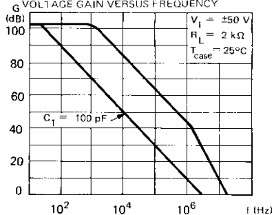
GAIN EN TENSION EN FONCTION DE LA FRE- QUENCE VOLTAGE GAIN VERSUS FREQUENCY
