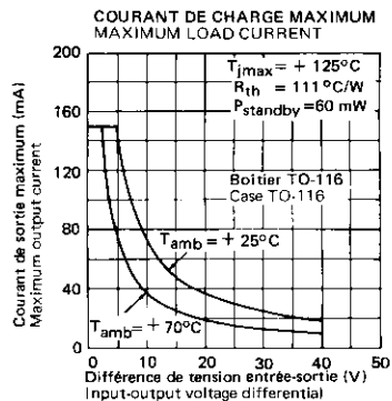
CARACTÉRISTIQUES DE REGULATION AVEC LIMITATION DE COURANT LOAD REGULATION WITH CURRENT LIMITING
