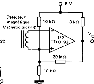
AMPLIFICATEUR TRANSCONDUCTEUR TRANSDUCER AMPLIFIER
