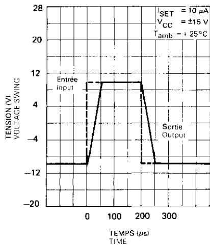
AMPLIFICATEUR SUIVEUR REPONSE EN IMPULSION VOLTAGE FOLLOWER PULSE RESPONSE
