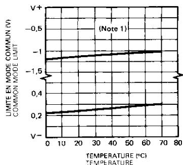
LIMITES EN MODE COMMUN COMMON MODE LIMITS
