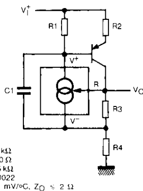
Fig. 6. - Thermomètre à basse impédance de sortie.
