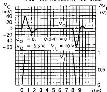
Fig. 12 — REPONSE TRANSITOIRE EN TENSION VOLTAGE TRANSIENT RESPONSE
