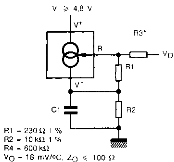
Fig. 5. - Thermomètre à basse impédance de sortie.
