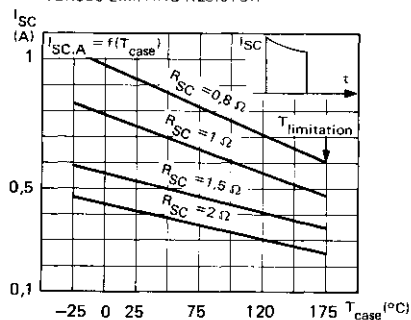
COURANT DE COURT-CIRCUIT EN FONCTION DE LA TEMPERATURE DE BOITIER SHORT-CIRCUIT CURRENT VERSUS CASE TEMPERATURE
