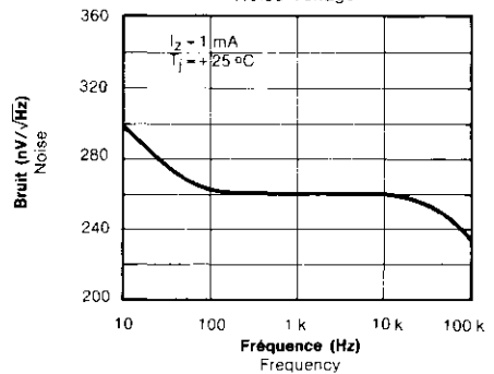
Tension de bruit Noise voltage
