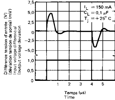
REPONSE TRANSITOIRE A UNE VARIATION DE LA TENSION D'ENTREE LINE TRANSIENT RESPONSE
