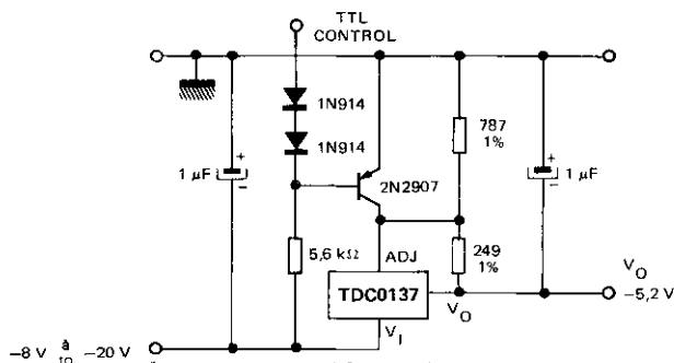
* Régulateur avec coupure électrique -5,2 V -5,2 V regulator with Electronic shutdown
