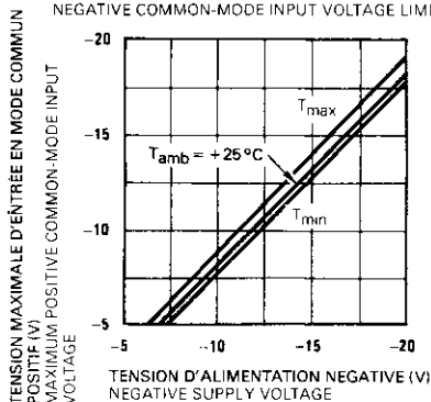
TENSION MAXIMALE D'ENTRÉE EN MODE COMMUN NEGATIF NEGATIVE COMMON-MODE INPUT VOLTAGE LIMIT
