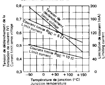
TENSION DE DECLENCHEMENT DE LA LIMITATION DE COURANT CURRENT LIMITING SENSE VOLTAGE
