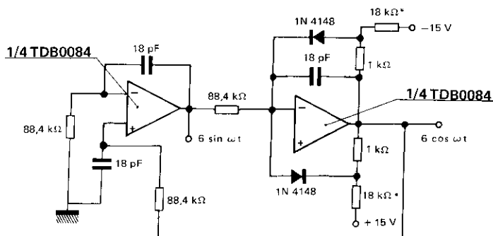
OSCILLATEUR A QUADRATURE QUADRATURE OSCILLATOR
