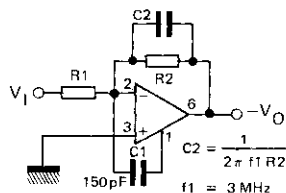
COMPENSATION AVEC BOUCLE D'AVANCE DE PHASE FEED FORWARD COMPENSATION
