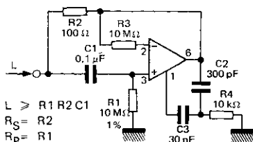
GENERATEUR D'ONDES SINUSOÏDALES SINE WAVE OSCILLATOR
