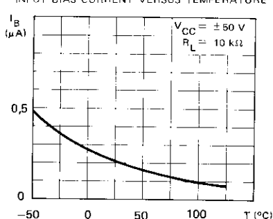
COURANT DE POLARISATION EN FONCTION DE LA TEMPERATURE INPUT BIAS CURRENT VERSUS TEMPERATURE
