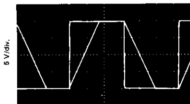
REPONSE IMPULSIONNELLE EN INVERSEUR INVERTER PULSE RESPONSE
