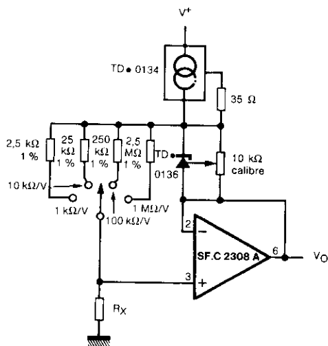
Figure 8. Ohmètre linéaire Linear Ohmmeter
