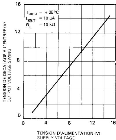
DYNAMIQUE DE SORTIE OUTPUT VOLTAGE SWING
