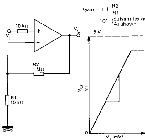
AMPLIFICATEUR SOMMEUR, TENSION CONTINUE DC SUMMING AMPLIFIER
