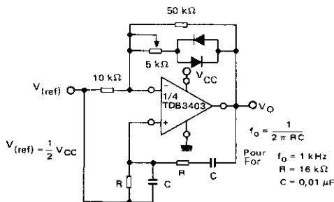
OSCILLATEUR A PONT DE WIEN WIEN BRIDGE OSCILLATOR
