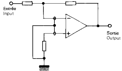
AMPLIFICATEUR INVERSEUR INVERTING AMPLIFIER
