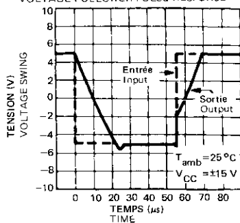
AMPLIFICATEUR SUIVEUR REPONSE EN IMPULSION VOLTAGE FOLLOWER PULSE RESPONSE
