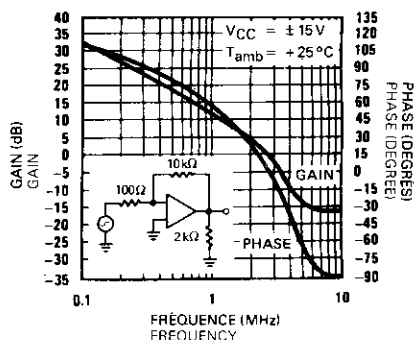
DIAGRAMME DE BODE (TDx 0149) BODE DIAGRAM
