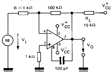
AMPLIFICATEUR INVERSEUR INVERTING AMPLIFIER
