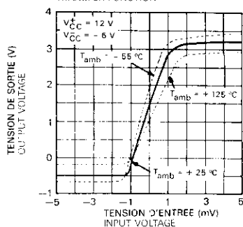
CARACTERISTIQUES DE TRANSFERT TRANSFER FUNCTION
