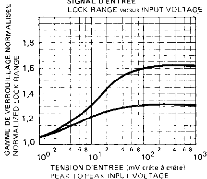
FIG. 5— GAMME DE VERROUILLAGE/ SIGNAL D'ENTRÉE LOCK RANGE versus INPUT VOLTAGE
