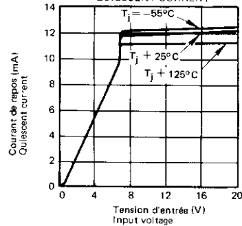
COURANT DE REPOS QUIESCENT CURRENT
