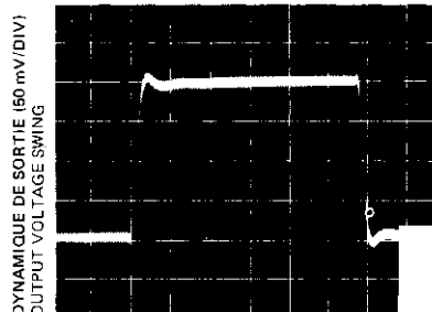
REPONSE A UNE IMPULSION DE FAIBLE AMPLITUDE (ENTREE NON INVERSEUSE) SMALL SIGNAL NON-INVERTING
