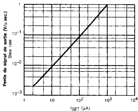
Fig. 2. - Pente maximale du signal de sortie pour un fonctionnement linéaire. Maximum slew rate for linear operation.
