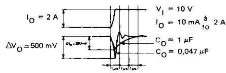
Fig. 10 — REPONSE TRANSITOIRE DANS LA CHARGE LOAD TRANSIENT RESPONSE
