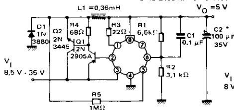
RÉGULATEUR DE TENSION A DÉCOUPAGE 4 A 4 A SWITCHING REGULATOR
