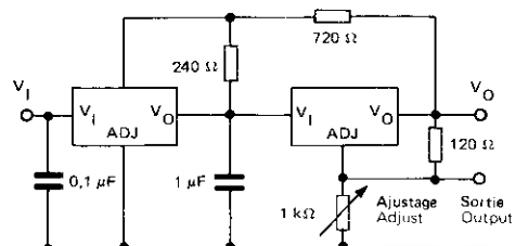
FIG.21 — REGULATEUR SUIVEUR TRACKING PRE REGULATOR
