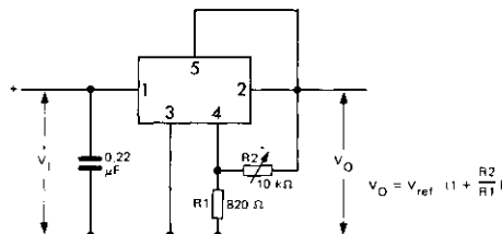
Fig. 19 — REGULATEUR DE TENSION PROGRAMMABLE PROGRAMMABLE VOLTAGE REGULATOR
