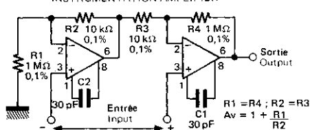
AMPLIFICATEUR DE MESURE INSTRUMENTATION AMPLIFIER
