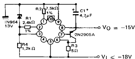
AMELIORATION DE LA REGULATION EN FONCTION DE LA TENSION D'ENTREE IMPROVING LINE REGULATION
