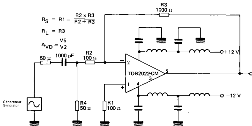
FIGURE 7: AMPLIFICATEUR INVERSEUR INVERTING AMPLIFIER
