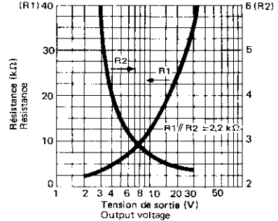
VALEUR OPTIMUM DU PONT DIVISEUR OPTIMUM DIVIDER RESISTANCE VALUE
