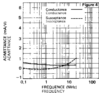
ADMITTANCE D'ENTREE SORTIE ( G_{11} ) EN CIRCUIT OUVERT INPUT ADMITTANCE WITH O/C OUTPUT
