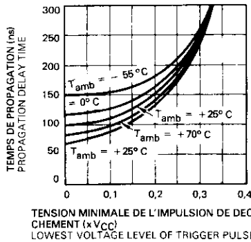
TEMPS DE PROPAGATION/AMPLITUDE DE L'IMPULSION DE DÉCLENCHEMENT PROPAGATION DELAY/VOLTAGE LEVEL OF TRIGGER PULSE
