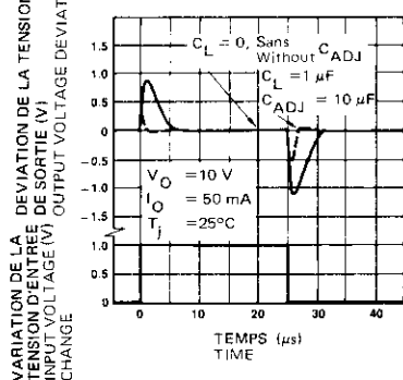
FIG. 13 — REPONSE TRANSITOIRE A UNE VARIATION DE LA TENSION D'ENTREE LINE TRANSIENT RESPONSE
