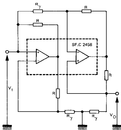
GYRATEUR GYRATOR
