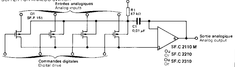
CIRCUIT INTERMEDIAIRE POUR COMMUTATEUR ANALOGIQUE BUFFER FOR ANALOG SWITCH
