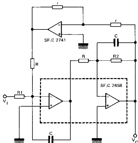
FILTRE PASSE BAS LOW-PASS FILTER
