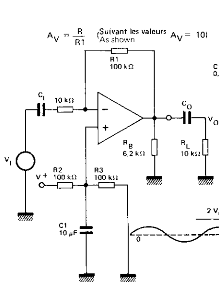
AMPLIFICATEUR INVERSEUR-LIAISON ALTERNATIVE AC COUPLED INVERTING AMPLIFIER
