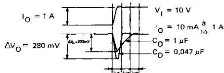
Fig. 9 — REPONSE TRANSITOIRE DANS LA CHARGE LOAD TRANSIENT RESPONSE
