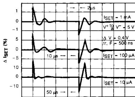
Fig. 4. - Réponse transitoire. Transient response.
