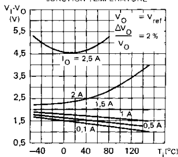
Fig. 13 - TENSION DIFFERENTIELLE "ENTREE-SORTIE" EN FONCTION DE LA TEMPERATURE DE JONCTION DROP-OUT VOLTAGE VERSUS JUNCTION TEMPERATURE
