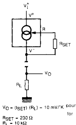
Fig. 5. - Thermomètre à basse impédance de sortie.
