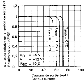
CARACTÉRISTIQUES DE LIMITATION DE COURANT CURRENT LIMITING CHARACTERISTICS
