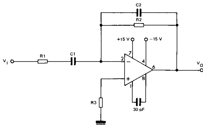
DIFFÉRENTIATEUR SIMPLE PRACTICAL DIFFENTIATOR
