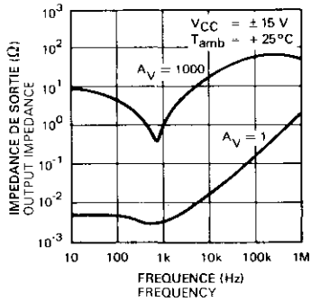
IMPEDANCE DE SORTIE EN BOUCLE FERMÉE CLOSED LOOP OUTPUT IMPEDANCE
