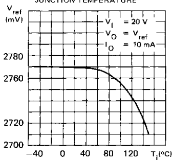
Fig. 7 — TENSION DE REFERENCE EN FONCTION DE LA TEMPERATURE DE JONCTION REFERENCE VOLTAGE VERSUS JUNCTION TEMPERATURE
