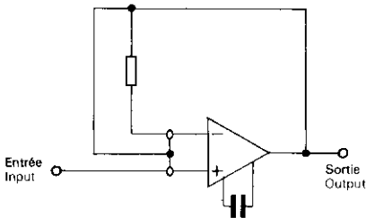
AMPLIFICATEUR SUIVEUR FOLLOWER AMPLIFIER
