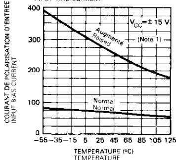
COURANT DE POLARISATION D'ENTREE INPUT BIAS CURRENT
