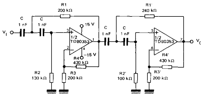
Filtre actif passe-haut du quatrième ordre (BUTTERWORTH) Fourth order high pass BUTTERWORTH filter
