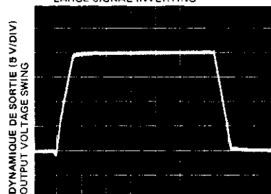
REPONSE A UNE IMPULSION DE FORTE AMPLITUDE (ENTREE INVERSEUSE) LARGE SIGNAL INVERTING
