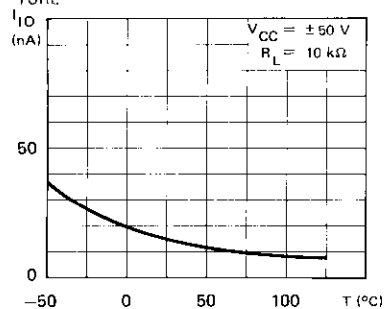
COURANT DE DÉCALAGE À L'ENTRÉE EN FONCTION DE LA TEMPERATURE INPUT OFFSET CURRENT VERSUS TEMPERA- TURE
