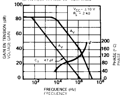
REPONSE EN FREQUENCE EN BOUCLE OUVERTE OPEN LOOP FREQUENCY RESPONSE
