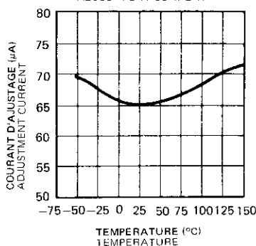
COURANT D'AJUSTAGE ADJUSTMENT CURRENT
