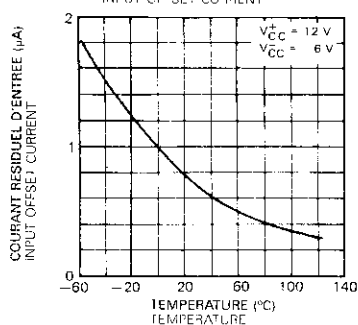
COURANT RESIDUEL D'ENTREE INPUT OFFSET CURRENT
