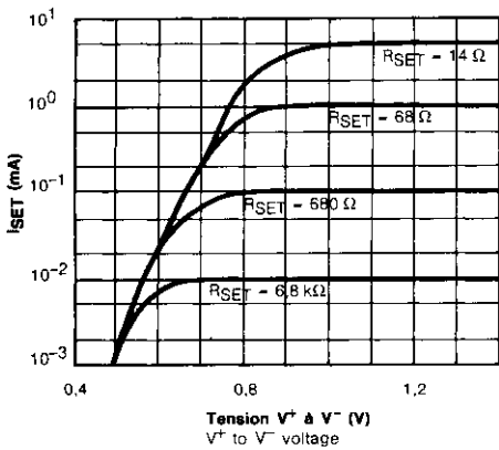
Fig. 7. - Tension d'établissement. Turn-on voltage.
