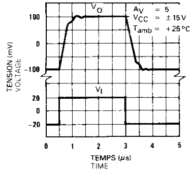
VITESSE DE MONTÉE SLEW RATE
