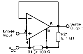
AUGMENTATION DE L'EXCURSION NEGATIVE SOUS CHARGE INCREASING NEGATIVE SWING UNDER LOAD
