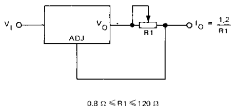
FIG. 2— SOURCE DE COURANT DE PRECISION PRECISION CURRENT LIMITER
