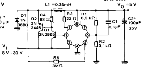
RÉGULATEUR DE TENSION A DÉCOUPAGE 2 A 2 A SWITCHING REGULATOR
