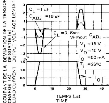
FIG. 14 — REPONSE TRANSITOIRE A UNE VARIATION DE CHARGE LOAD TRANSIENT RESPONSE
