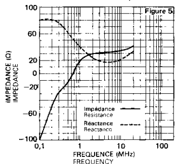
IMPEDANCE DE SORTIE, ( G_{22} ) ENTREE EN COURT-CIRCUIT OUTPUT IMPEDANCE WITH S/C INPUT
