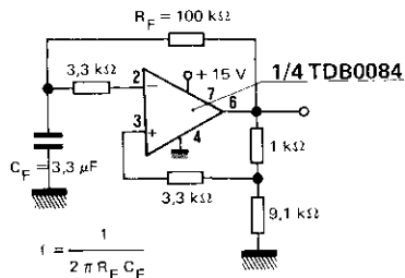
AMPLIFICATEUR DE DISTRIBUTION AUDIO AUDIO DISTRIBUTION AMPLIFIER
