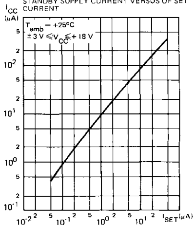
COURANT D'ALIMENTATION EN FONCTION DU COURANT DE REGLAGE STANDBY SUPPLY CURRENT VERSUS OF SET CURRENT
