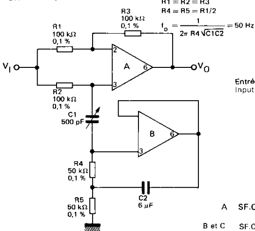
CIRCUIT INTERMEDIAIRE POUR COMMUTATEUR ANALOGIQUE BUFFER FOR ANALOG SWITCH
