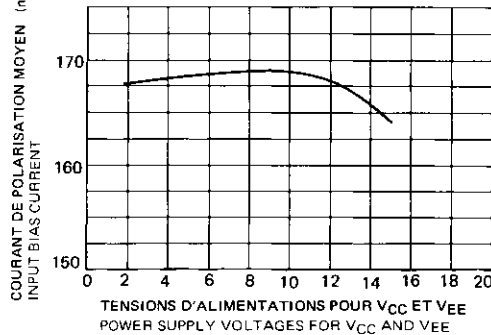
COURANT DE POLARISATION MOYEN EN FONCTION DE LA TENSION D'ALIMENTATION INPUT BIAS CURRENT VERSUS SUPPLY VOLTAGE
