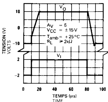
RÉPONSE A UNE IMPULSION DE FORTE AMPLITUDE (TDx 0148) LARGE SIGNAL PULSE RESPONSE
