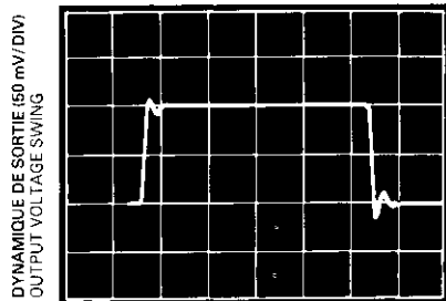
REPONSE A UNE IMPULSION DE FAIBLE AMPLITUDE TDC 0155 A_V = +1 SMALL SIGNAL PULSE RESPONSE
