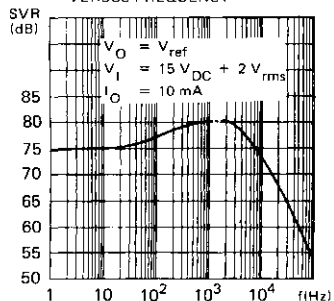
Fig. 11 — TAUX DE REJECTION DU AUX ALIMENTATIONS EN FONCTION DE LA FREQUENCE SUPPLY VOLTAGE REJECTION RATIO VERSUS FREQUENCY
