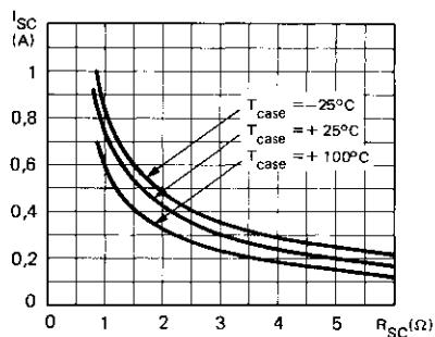
COURANT DE COURT-CIRCUIT CRETE EN FONCTION DE LA RESISTANCE DE LIMITATION PEAK SHORT-CIRCUIT OUTPUT CURRENT VERSUS LIMITING RESISTOR
