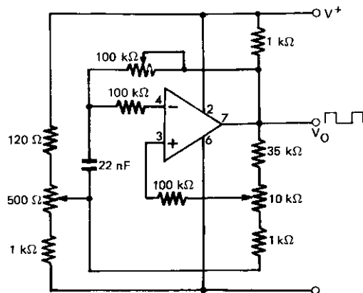
GENÉRATEUR D'IMPULSIONS PULSE GENERATOR
