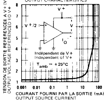
CARACTERISTIQUES DE SORTIE OUTPUT CHARACTERISTICS
