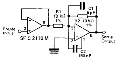
CONVERTISSEUR RAPIDE * AC/DC FAST AC/DC CONVERTER
