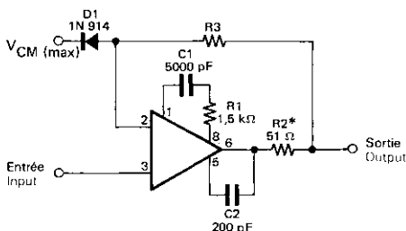
AMPLIFICATEUR SUIVEUR VOLTAGE FOLLOWER
