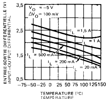
TENSION DIFFÉRENTIELLE DIFFERENTIAL VOLTAGE
