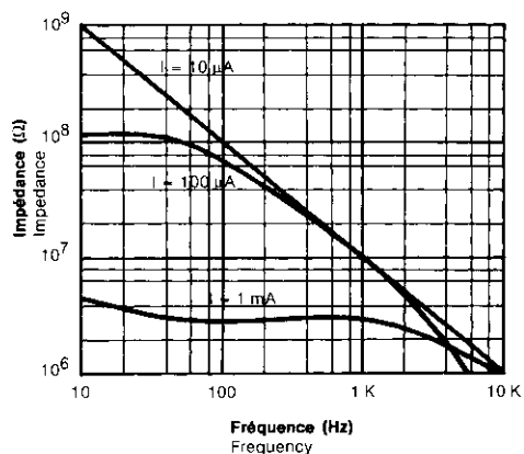
Fig. 1. - Impédance de sortie. Output impedance.
