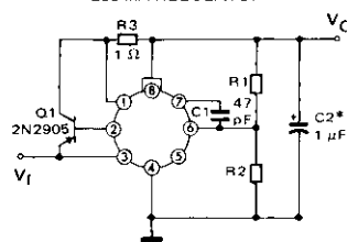
REGULATEUR 200 mA 200 mA REGULATOR
