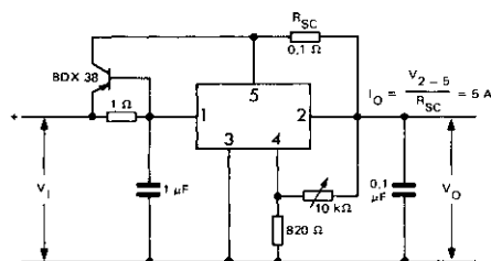
Fig. 22 — REGULATEUR DE TENSION A FORT COURANT AVEC PROTECTION CONTRE LES COURTS- CIRCUITS HIGH CURRENT VOLTAGE REGULATOR WITH SHORT CIRCUIT PROTECTION
