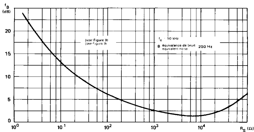
FIGURE 10: FACTEUR DE BRUIT NOISE FIGURE
