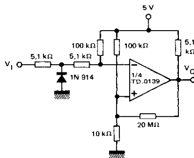
DETECTEUR DE PASSAGE A ZERO ZERO CROSSING DETECTOR
