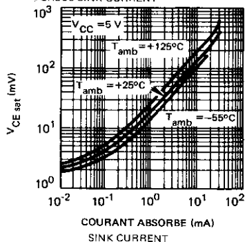
TENSION DU TRANSISTOR DE DECHARGE EN FONCTION DU COURANT ABSORBE DISCHARGE TRANSISTOR VOLTAGE VERSUS SINK CURRENT
