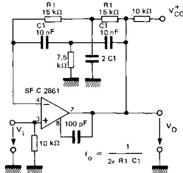
AMPLIFICATEUR SELECTIF SELECTIVE AMPLIFIER
