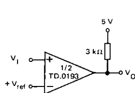
MONTAGE CLASSIQUE DU COMPAREUR BASIC COMPARETOR
