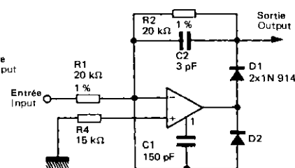
REDRESSEUR RAPIDE DEMI-ALTERNANCE FAST HALF WAVE RECTIFIER
