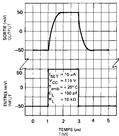
AMPLIFICATEUR SUIVEUR REPONSE TRANSITOIRE VOLTAGE FOLLOWER TRANSIENT RESPONSE
