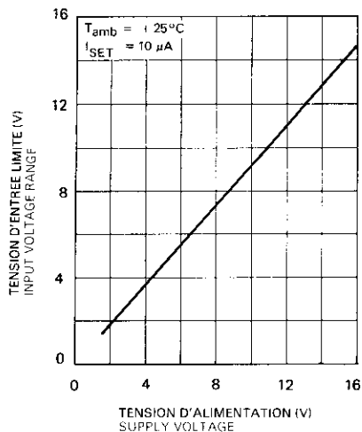
TENSION D'ENTREE LIMITE INPUT VOLTAGE RANGE
