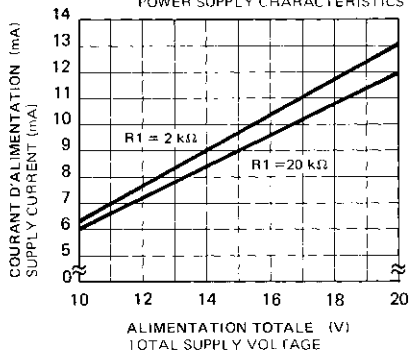
FIG. 3— CARACTERISTIQUES DE L'ALIMENTATION MENTATION POWER SUPPLY CHARACTERISTICS
