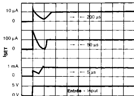
Fig. 3. - Démarrage (mise en route) Start up
