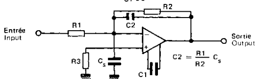
COMPENSATION DES CAPACITES PARASITES D'ENTREE COMPENSATING FOR STRAY INPUT CAPACITANCES
