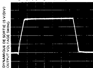
REPONSE A UNE IMPULSION DE FORTE AMPLITUDE (ENTREE INVERSEUSE) LARGE SIGNAL INVERTING
