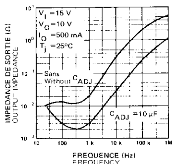
FIG. 12 — IMPEDANCE DE SORTIE OUTPUT IMPEDANCE
