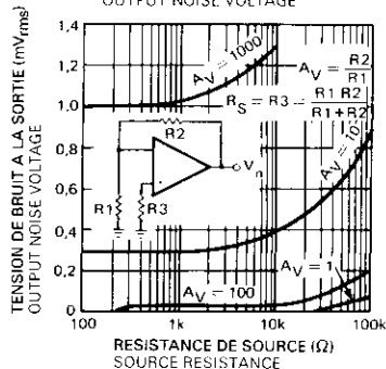
TENSION DE BRUIT A LA SORTIE OUTPUT NOISE VOLTAGE
