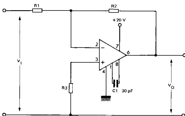
FONCTIONNEMENT SANS ALIMENTATION NÉGATIVE OPERATING WITHOUT A NEGATIVE SUPPLY
