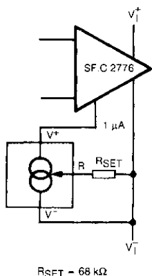
Fig. 7. - Polarisation de faible puissance. Micropower bias.
