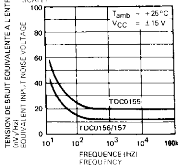
TENSION DE BRUIT EQUIVALENTE A L'ENTREE EQUIVALENT INPUT NOISE VOLTAGE
