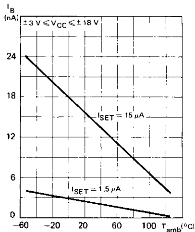
COURANT DE POLARISATION D'ENTREE INPUT BIAS CURRENT
