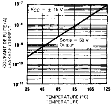
COURANT DE FUITE EN FONCTION DE LA TEMPÉRATURE LEAKAGE CURRENT VERSUS TEMPERATURE
