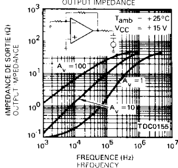
IMPEDANCE DE SORTIE OUTPUT IMPEDANCE
