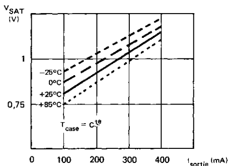
TENSION DE SATURATION EN FONCTION DU COURANT DE SORTIE SATURATION VOLTAGE VERSUS OUTPUT CURRENT
