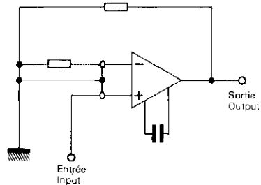
AMPLIFICATEUR NON-INVERSEUR NON-INVERTING AMPLIFIER
