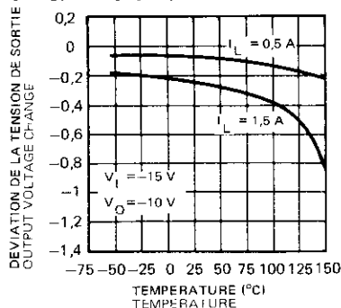
REGULATION EN FONCTION DE LA CHARGE LOAD REGULATION
