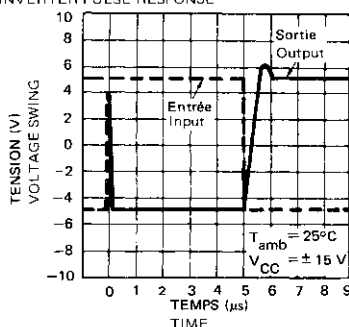
AMPLIFICATEUR INVERSEUR REPONSE EN IMPULSION INVERTER PULSE RESPONSE
