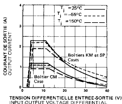
FIG. 4 — LIMITATION DE COURANT CURRENT LIMIT
