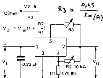
Fig. 20 — REGULATEUR DE TENSION PROGRAMMABLE AVEC LIMITATION DE COURANT PROGRAMMABLE VOLTAGE REGULATOR WITH CURRENT LIMITING
