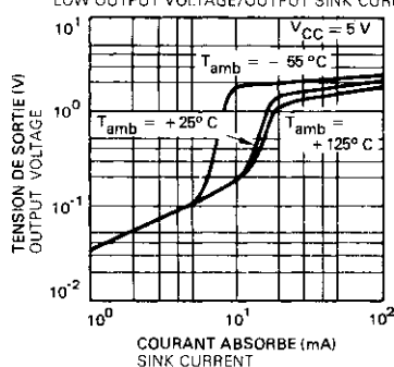
TENSION DE SORTIE (ETAT BASI)/ COURANT ABSORBE A LA SORTIE LOW OUTPUT VOLTAGE/OUTPUT SINK CURRENT
