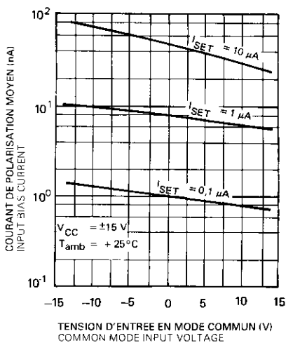
COURANT DE POLARISATION MOYEN INPUT BIAS CURRENT
