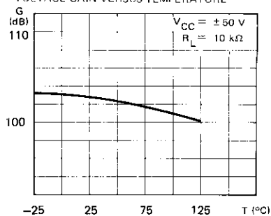
GAIN EN TENSION EN FONCTION DE LA TEM- PERATURE VOLTAGE GAIN VERSUS TEMPERATURE
