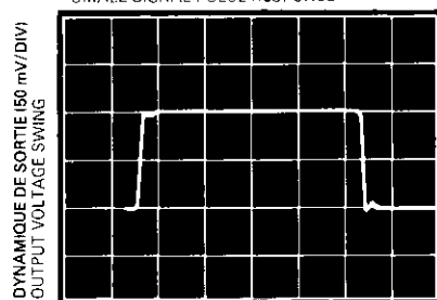
REPONSE A UNE IMPULSION DE FAIBLE AMPLITUDE TDC 0156 A_V = +1 SMALL SIGNAL PULSE RESPONSE
