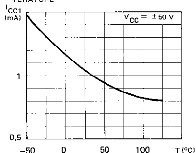
COURANT D'ALIMENTATION POSITIF EN FON- CTION DE LA TEMPERATURE POSITIVE SUPPLY CURRENT VERSUS TEM- PERATURE
