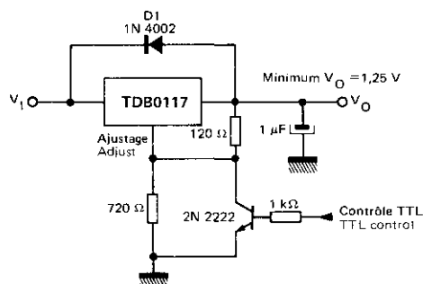
FIG.19 — REGULATEUR 5 V AVEC COUPEURE ELECTRONIQUE 5 V ELECTRONIC SHUT DOWN REGULATOR
