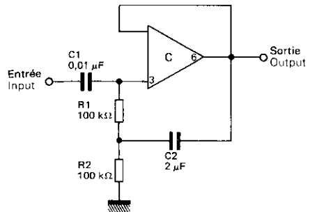
AMPLIFICATEUR ALTERNATIF A IMPEDANCE D'ENTREE ELEVÉE HIGH INPUT IMPEDANCE AC AMPLIFIER
