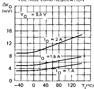
Fig. 8 — REGULATION EN TENSION EN FONCTION DE LA CHARGE VOLTAGE LOAD REGULATION
