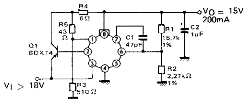
REGULATEUR DE TENSION AVEC REDUCTION AUTOMATIQUE DU COURANT DE COURT-CIRCUIT LINEAR REGULATOR WITH FOLDBACK CURRENT LIMITING
