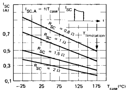
COURANT DE COURT-CIRCUIT EN FONCTION DE LA TEMPERATURE DE BOITIER SHORT-CIRCUIT CURRENT VERSUS CASE TEMPERATURE
