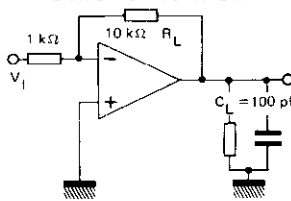
Fig.2 : AMPLIFICATEUR INVERSEUR A GAIN DE 10 GAIN-OF-10 INVERTING AMPLIFIER
