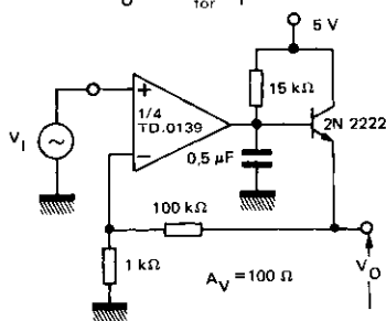
AMPLIFICATEUR OPERATIONNEL BASSE FREQUENCE LOW FREQUENCY OP AMP ( V_O = 0 V pour V_I = 0 V) (for V_I = 0 V)
