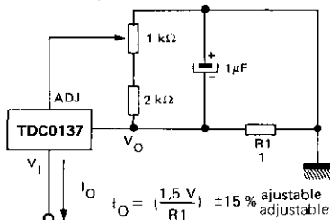
Régulateur de courant ajustable Adjustable current regulator
