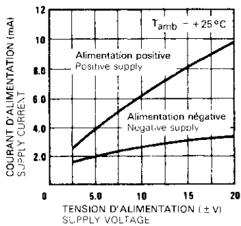
COURANT D'ALIMENTATION SUPPLY CURRENT
