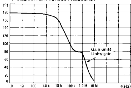
MARGE DE PHASE EN FONCTION DE LA FREQUENCE PHASE MARGIN VERSUS FREQUENCY
