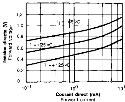
Caractéristiques directes Forward characteristics
