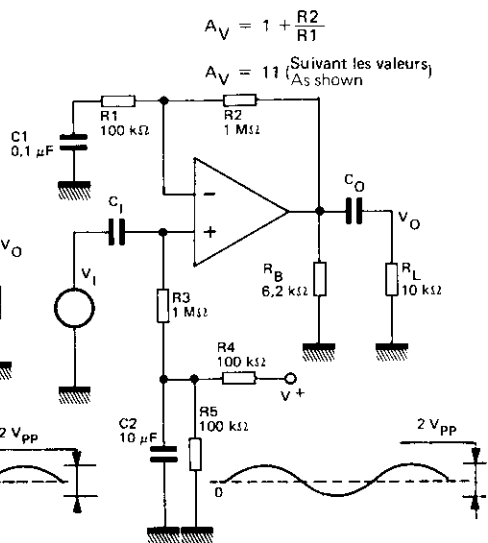
AMPLIFICATEUR NON-INVERSEUR-LIAISON ALTERNATIVE AC COUPLED NON INVERTING AMPLIFIER
