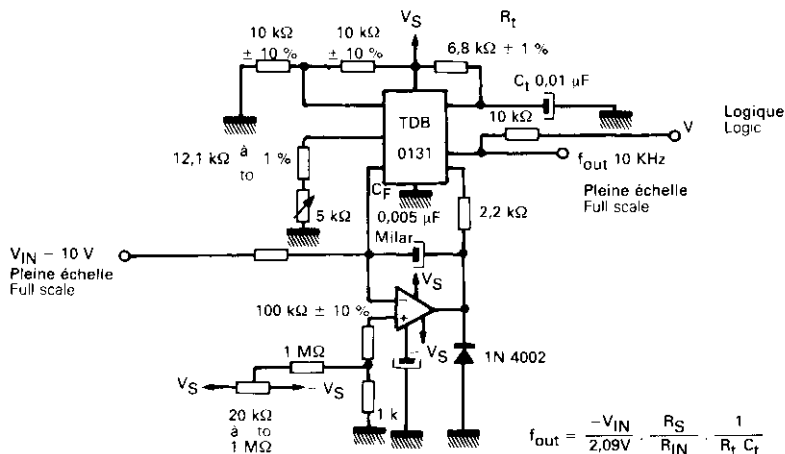
Figure 2 — Schéma simplifié du convertisseur tension-fréquence avec linéarité typique \pm 0,03 % ( f = 10 Hz à 11 KHz). Simple stand-alone voltage-to-frequency converter with \pm 0,03 % typical linearity ( f = 10 Hz to 11 KHz).
