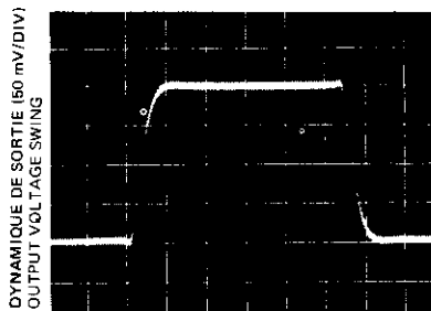
REPONSE A UNE IMPULSION DE FAIBLE AMPLITUDE (ENTREE INVERSEUSE) SMALL SIGNAL INVERTING
