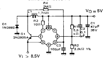
RÉGULATEUR A DÉCOUPAGE SWITCHING REGULATOR
