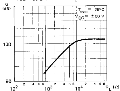
GAIN EN TENSION EN FONCTION DE R_L VOLTAGE GAIN VERSUS R_L
