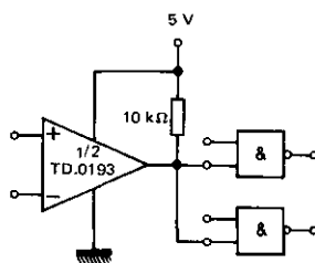
AMPLIFICATEUR TRANSCONDUCTEUR TRANSDUCER AMPLIFIER
