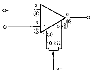
CONVERTISSEUR COURANT / TENSION CURRENT TO VOLTAGE CONVERTER
