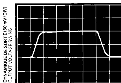
REPONSE A UNE IMPULSION DE FAIBLE AMPLITUDE TDC 0157 A_V = +5 SMALL SIGNAL PULSE RESPONSE
