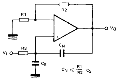
OPTIMISATION DU TEMPS DE REPOSE EN NEUTRALISANT LA CAPACITE D'ENTREE NEUTRALIZING INPUT CAPACITANCE TO OPTIMIZE RESPONSE TIME
