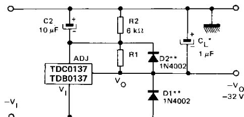
Régulateur négatif avec diodes de protection Negative regulator with protection diodes
