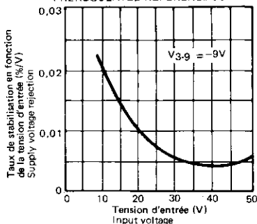
TAUX DE STABILISATION AVEC SOURCE DE POLARISATION PRERÉGLÉE SUPPLY VOLTAGE REJECTION WITH PREREGULATED REFERENCE SUPPLY
