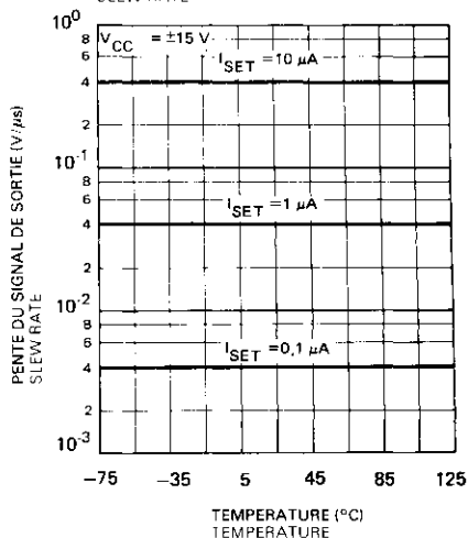
PENTE DU SIGNAL DE SORTIE SLEW RATE
