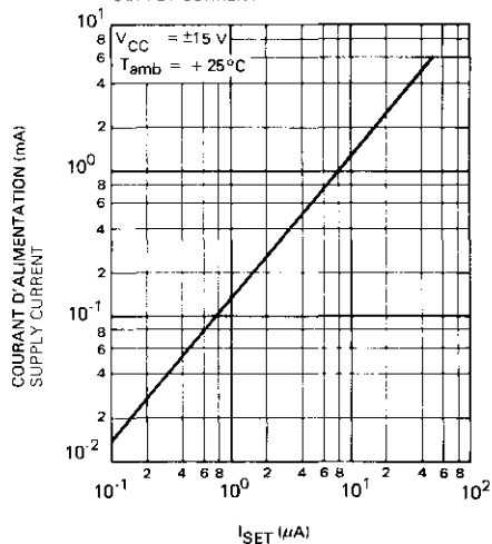
COURANT D'ALIMENTATION SUPPLY CURRENT
