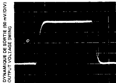
REPONSE A UNE IMPULSION DE FAIBLE AMPLITUDE (ENTREE INVERSEUSE) SMALL SIGNAL INVERTING
