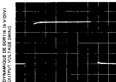
REPONSE A UNE IMPULSION DE FORTE AMPLITUDE (ENTREE NON INVERSEUSE) LARGE SIGNAL NON-INVERTING
