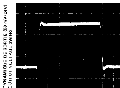
REPONSE A UNE IMPULSION DE FAIBLE AMPLITUDE (ENTREE NON INVERSEUSE) SMALL SIGNAL NON-INVERTING
