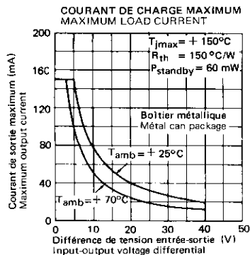
CARACTÉRISTIQUES DE REGULATION SANS LIMITATION DE COURANT LOAD REGULATION WITHOUT CURRENT LIMITING
