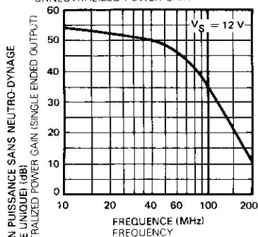
GAIN EN PUISSANCE SANS NEUTRO-DYNAGE UNNEUTRALIZED POWER GAIN
