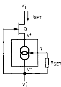
Fig. 10. - Adjonction d'un FET pour réduction de la capacité de shunt. FET cascading for low capacitance.
