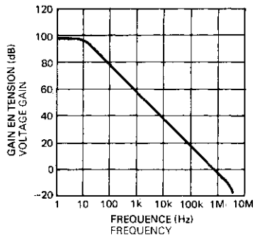
REPONSE EN FREQUENCE EN BOUCLE OUVERTE (TYP.) OPEN LOOP FREQUENCY RESPONSE
