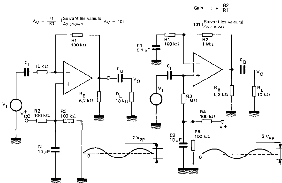
AMPLIFICATEUR INVERSEUR - LIAISON ALTERNATIVE ACCOUPLED INVERTING AMPLIFIER
