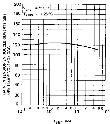
GAIN EN TENSION EN BOUCLE OUVERTE OPEN LOOP VOLTAGE GAIN
