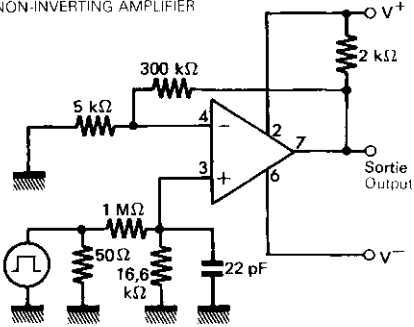
AMPLIFICATEUR NON INVERSEUR NON-INVERTING AMPLIFIER
