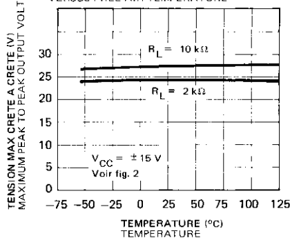
TENSION DE SORTIE MAX CRETE A CRETE EN FONCTION DE LA TEMPERATURE AMBIANTE MAXIMUM PEAK TO PEAK OUTPUT VOLTAGE VERSUS FREE-AIR TEMPERATURE
