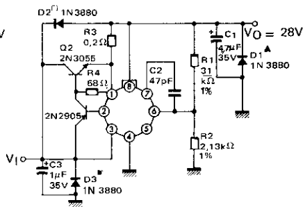
REGULATEUR DE TENSION 1 A AVEC DIODES DE PROTECTION 1 A REGULATOR WITH PROTECTIVE DIODES
