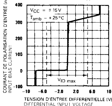
CARACTERISTIQUES D'ENTREE INPUT CHARACTERISTICS
