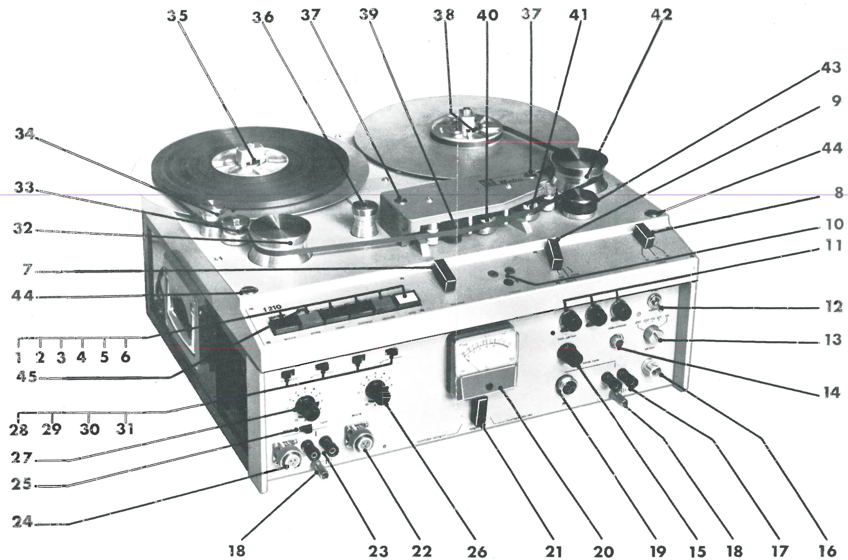
MAGNETOPHONE MONAURAL F 210 Vue d'ensemble repérée
