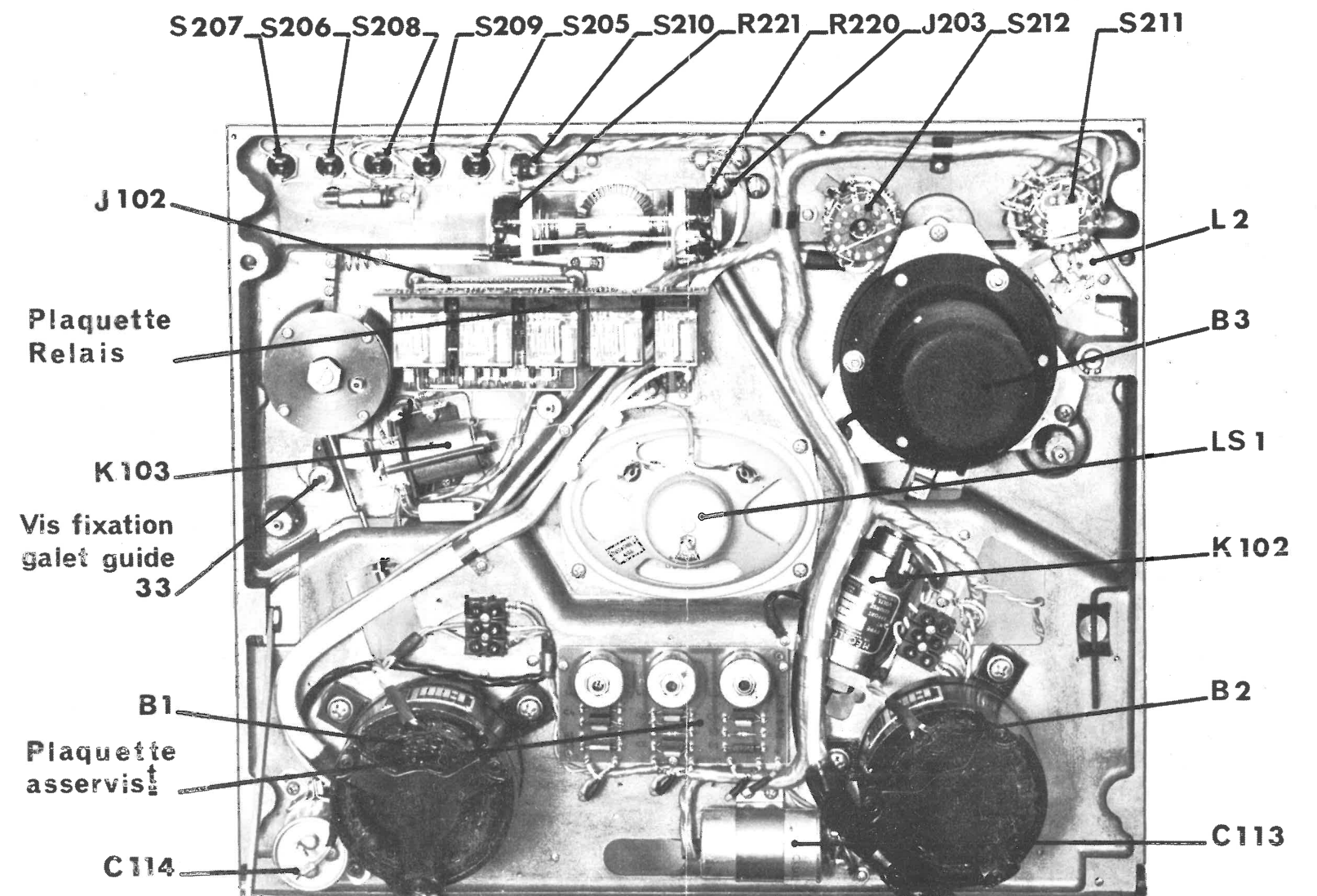
MAGNETOPHONE MONAURAL F 210 - Platine mécanique A1 Vue de dessous
