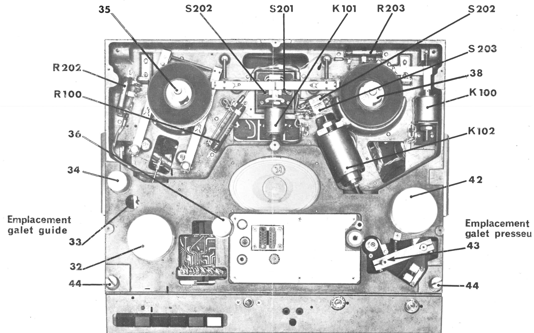
MAGNETOPHONE MONAURAL F 210 - Vue de dessus platine A1 (contre platine et bloc têtes déposés)
