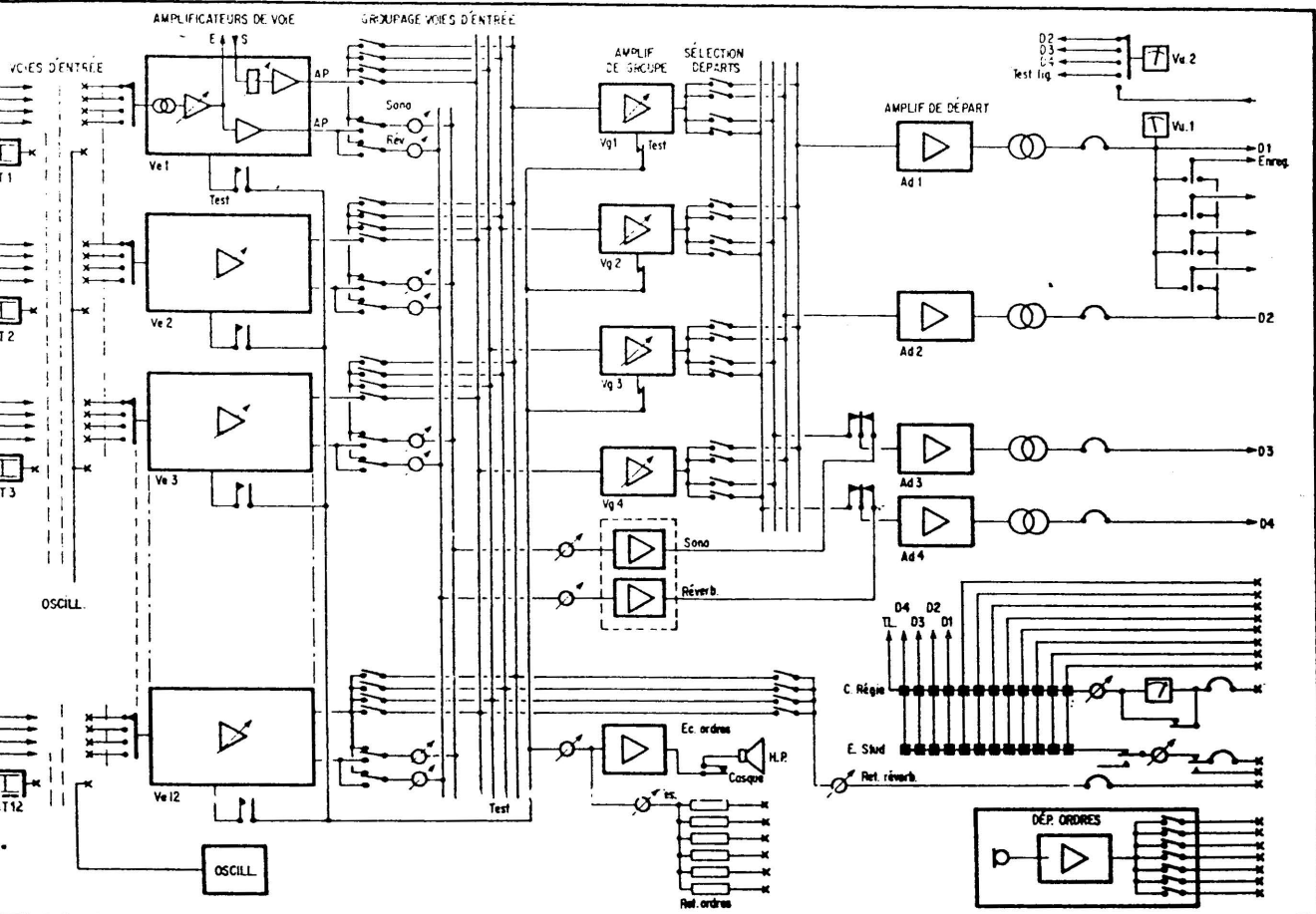
Fig. 4-25. — Schéma synoptique de la console UPS 2104 Schlumberger.
