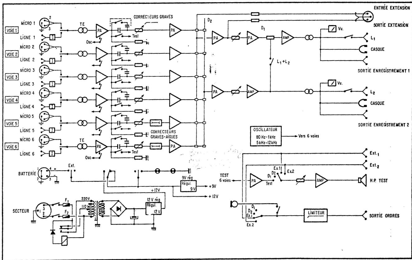
Fig. 4-23. — Schéma synoptique de l'unité de prise de son UPS 1602 Schlumberger.
