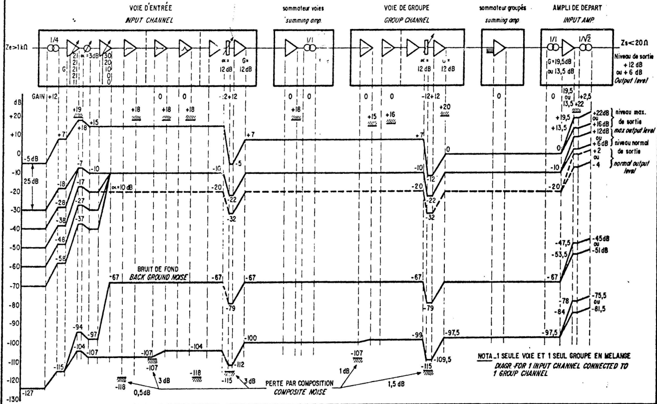
Fig. 4-32. — Diagramme des niveaux de la console UPS 4000 Schlumberger .
